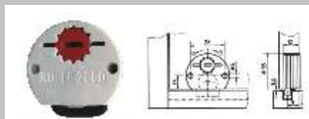
Rola inferioara alba Art. Nr. 684 562 100 Rola inferioara maro Art. Nr. 684 562 101
