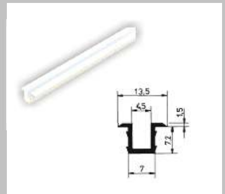
Profil de rulare PVC 3 m alb Art. Nr. 684 562 104 Profil de rulare PVC 3 m maro Art. Nr. 684 562 105 Profil de rulare PVC 3 m negru Art. Nr. 684 562 106 Profil de rulare PVC 3 m gri Art. Nr. 684 562 107
