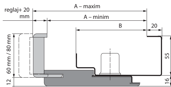
SECȚIUNE TOC PROIECT PREMIUM
