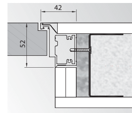
falț ascuns (deschidere spre interior)
