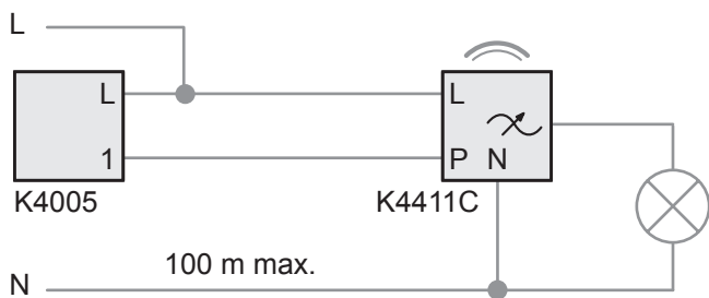
Schemă cu butoane de comandă la distanță
