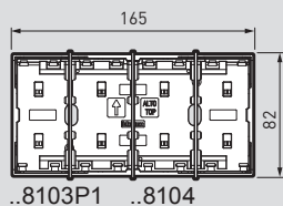
Ramă electrificată de 3+1 module, 4 module
