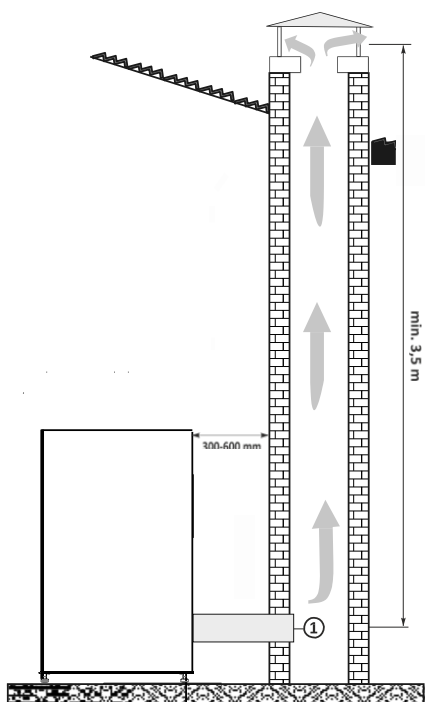
Schema 1. Racordarea Termosemineului pe peleți la coș
