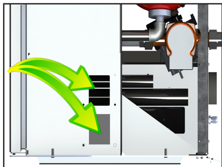
Schemă 9. Curățarea funinginii de pe țevile de fum prin orificiile de vizitare din ambele părți, în partea de jos a sobei - pasul 1
