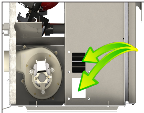
Schemă 10. Curățarea funinginii de pe țevile de fum prin orificiile de vizitare din ambele părți, în partea de jos a sobei - pasul 2
