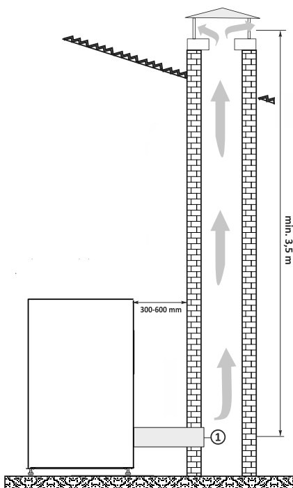
Schemă 1. Racordarea sobei pe peleți la coș
