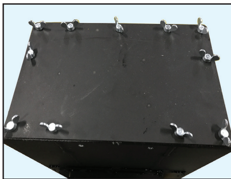
Schemă 7. Demontarea capacului pentru țevile de fum-1
