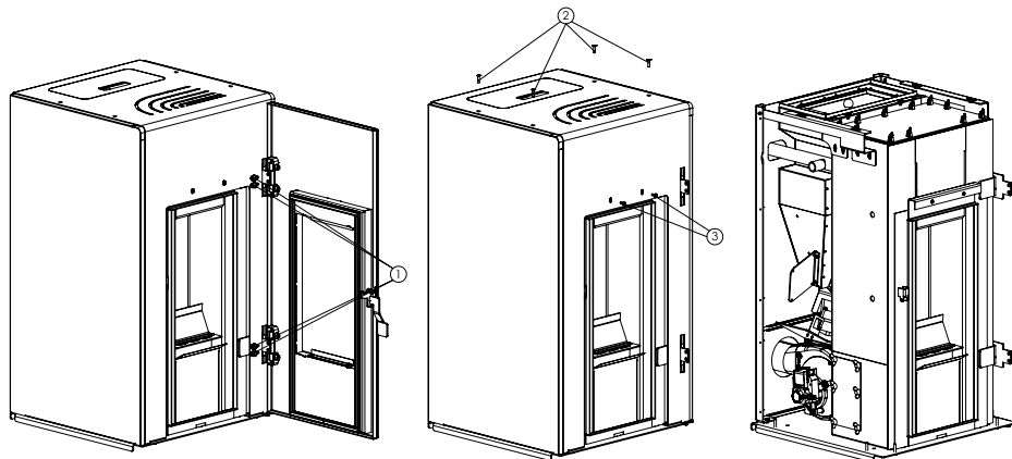
Schemă 6. Demontarea capacului pentru țevile de fum
