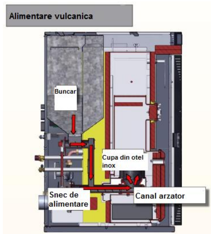
Figura 3. Alimentare vulcanica, cu combustibil
