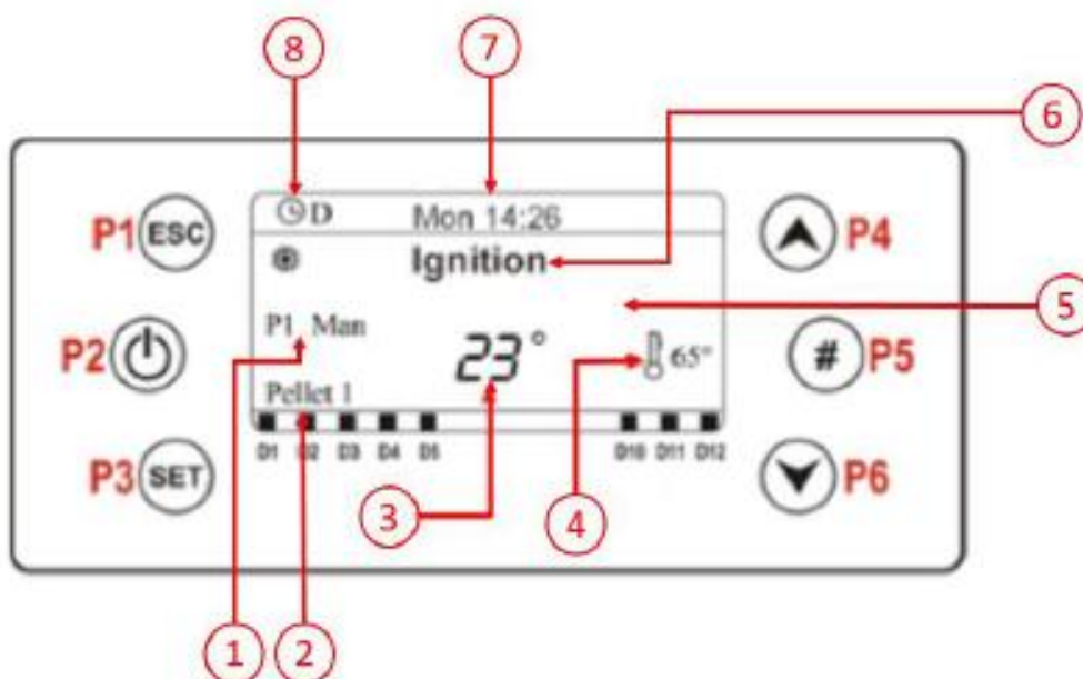
Figura 18. Display-ul LCD 100
