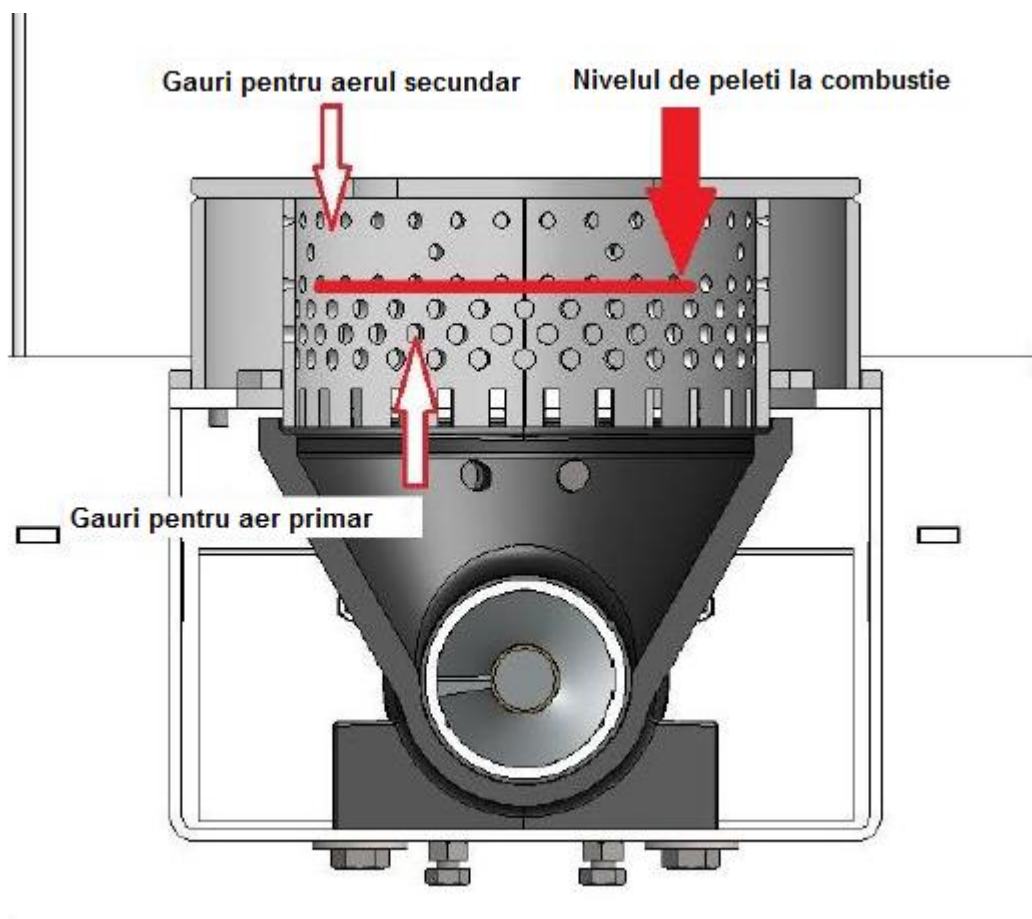
Figura 4. Combustia peletilor in creuzetul cromat
