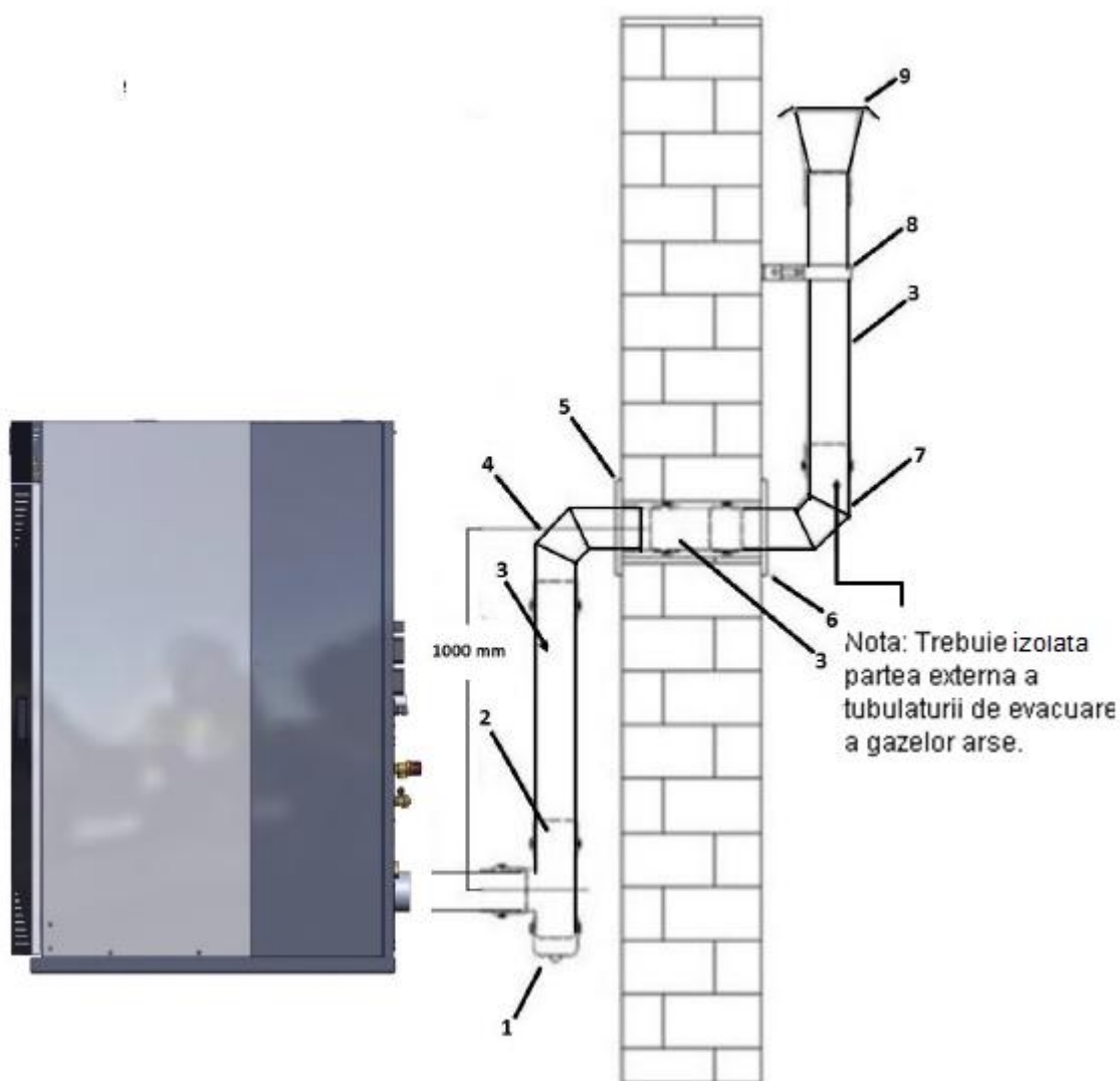
Figura 12. Instalarea tubulaturii de evacuare gaze arse
