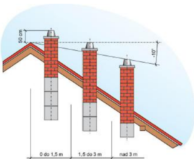
Figura 14. Înălțimea cosului
