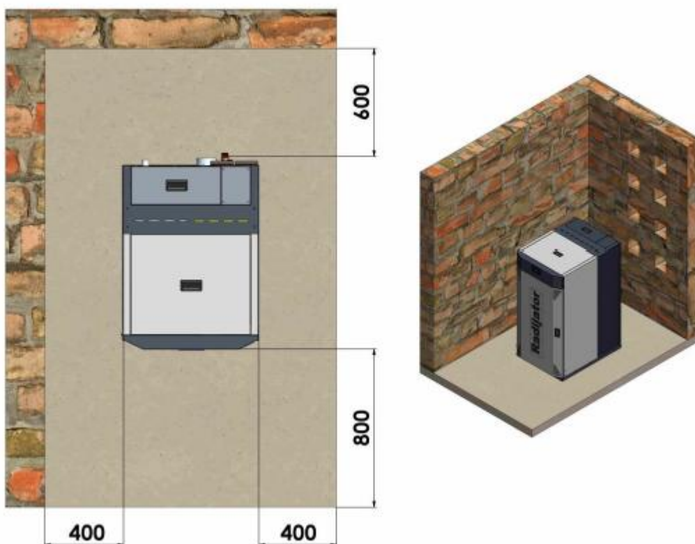
Figura 11 Amplasarea cazanului în centrala termică
