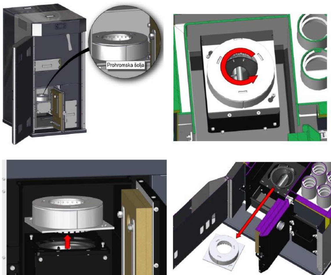
Figura 24. Demontarea creuzetului cromat cand se efectueaza curatarea
