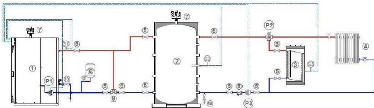
Figura 17. Schema hidraulica
