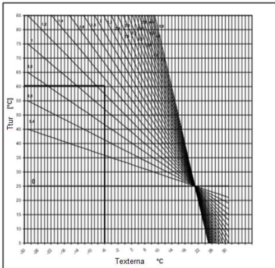
Figura 19. Senzor de temperatura externa
