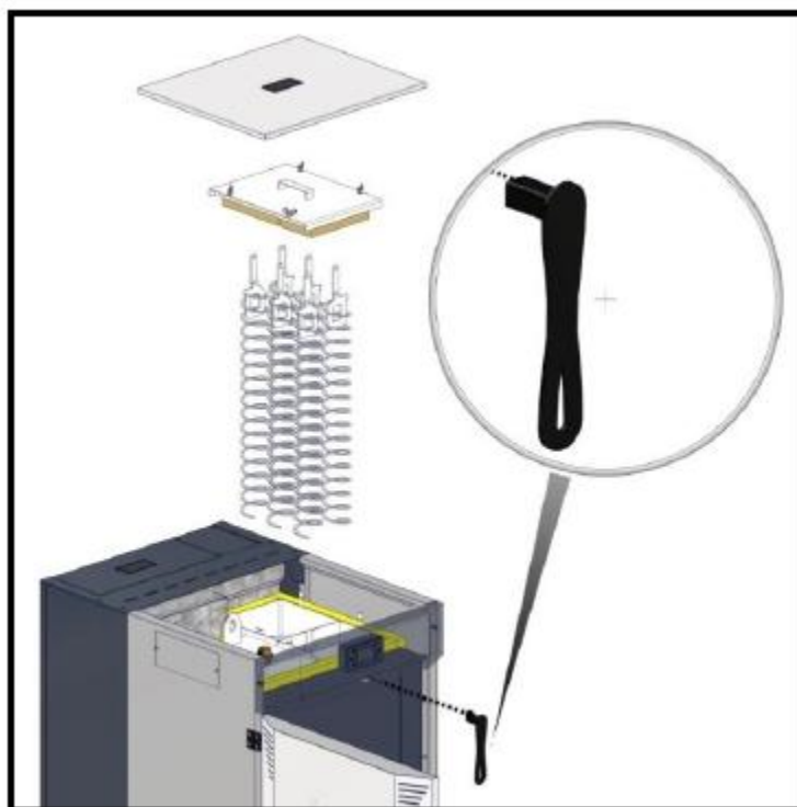
2. Turbulatoare
