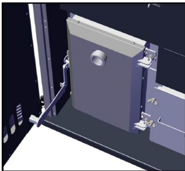
Figura 5. Deschiderea usii camerei de combustie
