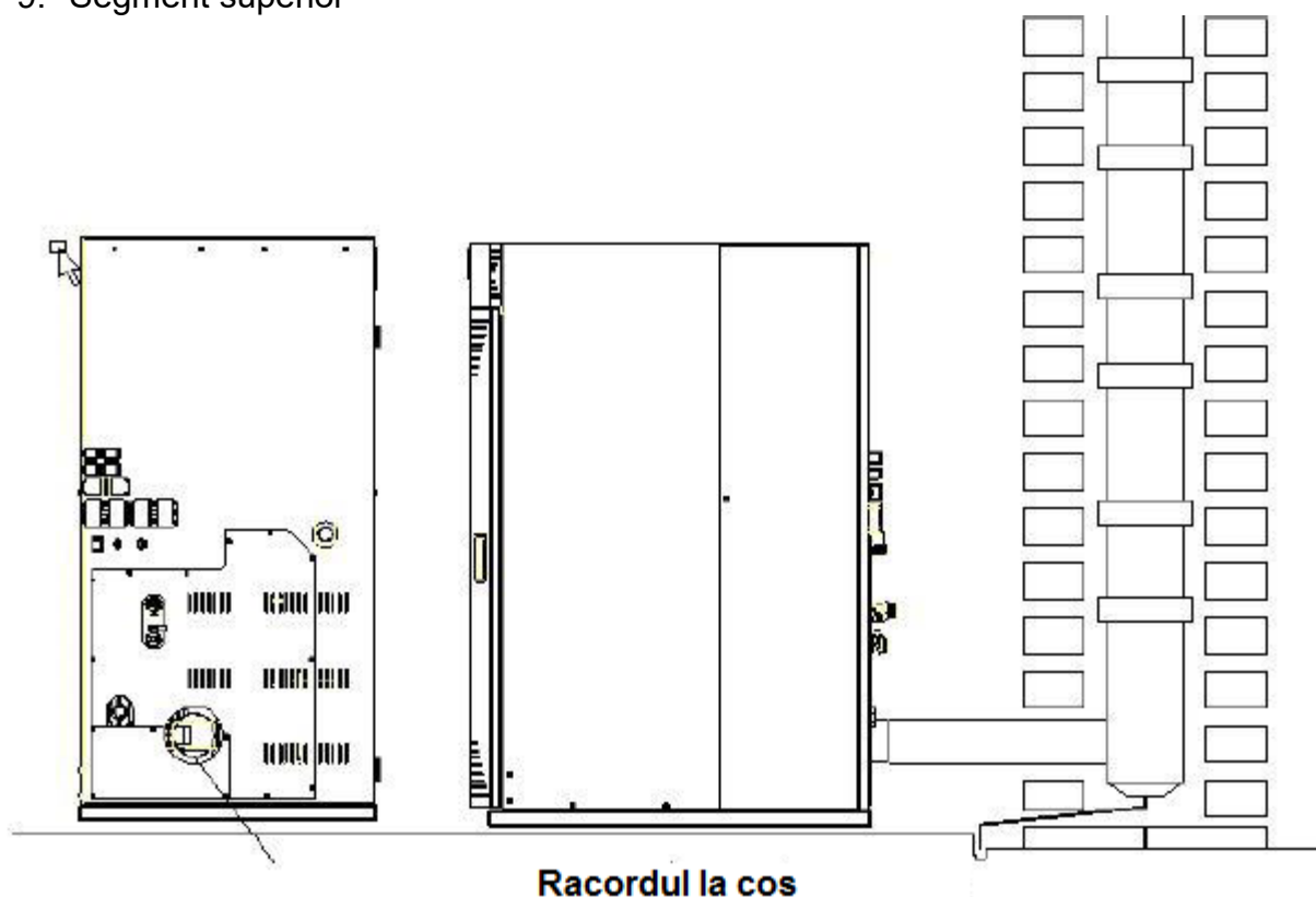
Figura 13. Racordul la cos
