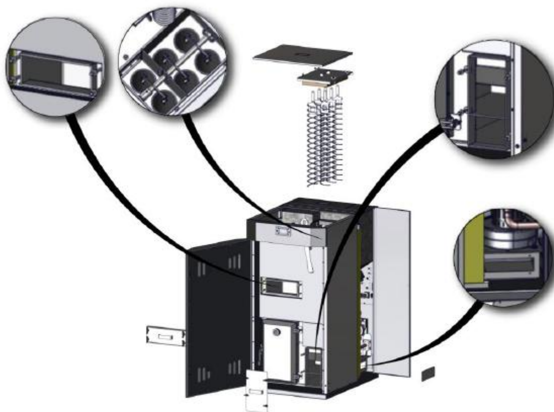
Figura 27. Orificiile de inspectie necesare pentru curatare
