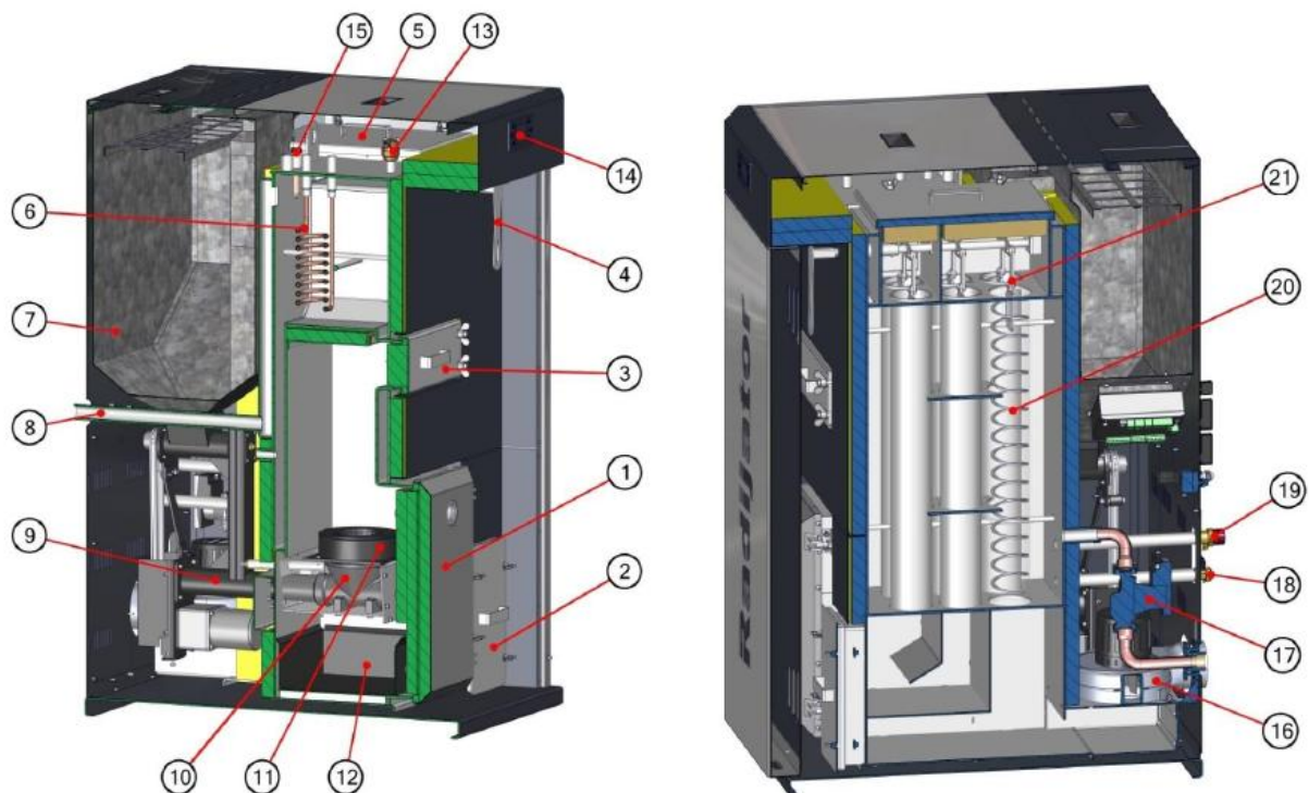
Figura 1. Setiunea cazanului Ecoflame Plus
