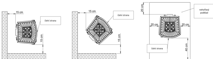
Obr. 3. Bezpečné vzdálenosti kotle od nehořlavých částí.
