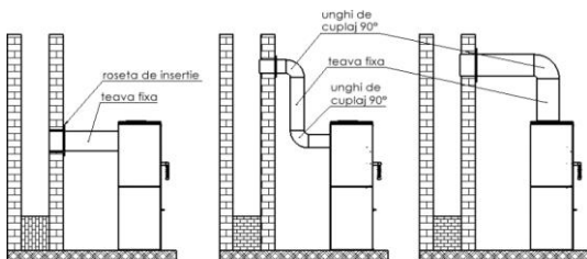
Fig.4. Schema de instalare a sobelor
