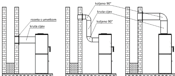
Crtež 4. Shematski prikaz priključivanja kaminske peći
