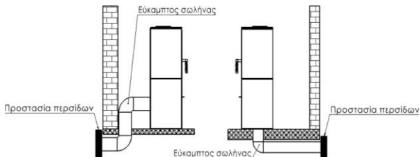
Σχ. 2. Διάγραμμα σύνδεσης παροχής αέρα
