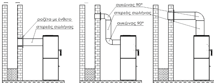
Σχ.4. Σχήμα σύνδεσης τζακιού
