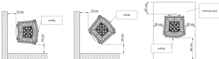
Joonis 3. Ahju ohutu kaugus mittesüttivatest osadest.
