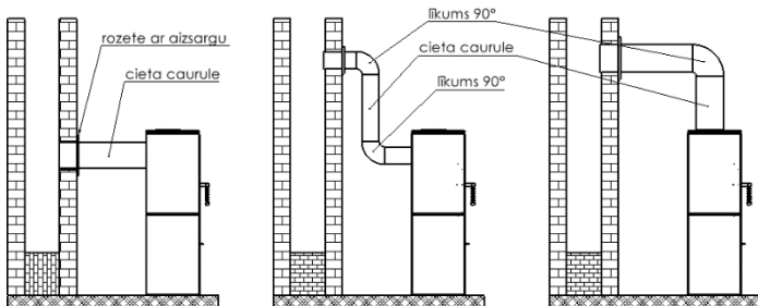
Att. 4 Kamīnkrāsns pievienošanas shēma
