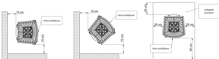
Att. 3. Droši plīts attālumumi no nedegošām daļām.
