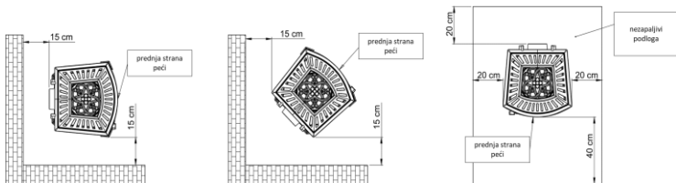
Crtež 3. Sigurne udaljenosti peći od nezapaljivih dijelova.
