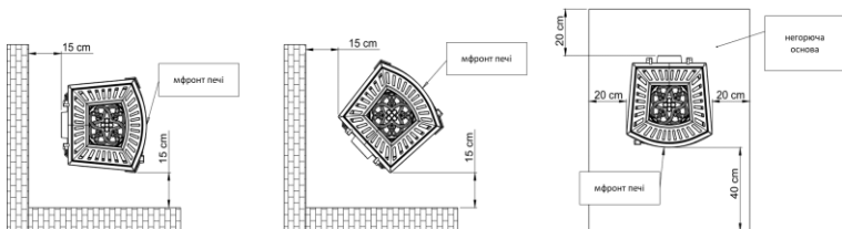
рис. 3. Безпечна відстань від печі до негорючих частин.
