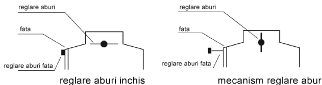
Fig. 5. Exemplu de reglare a aburilor
