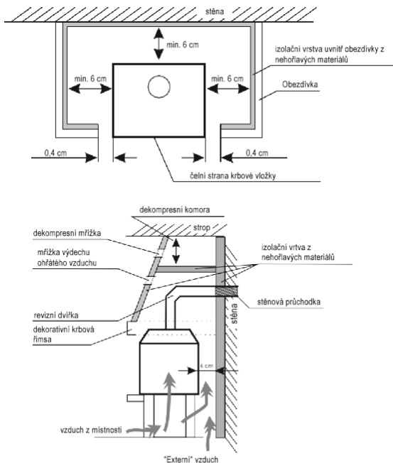
Obr. 3. Příklad montáže krbových vložek - pohled shora a z boku.
