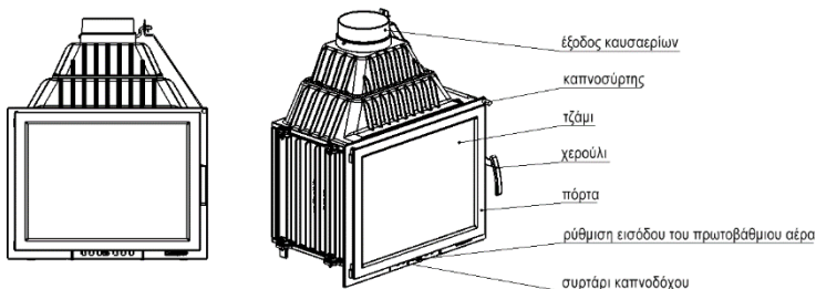
Σχ. 1. Σχήμα ενθέτου τζακιού.
