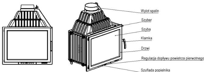
Rys. 1. Schemat wkładu kominkowego
