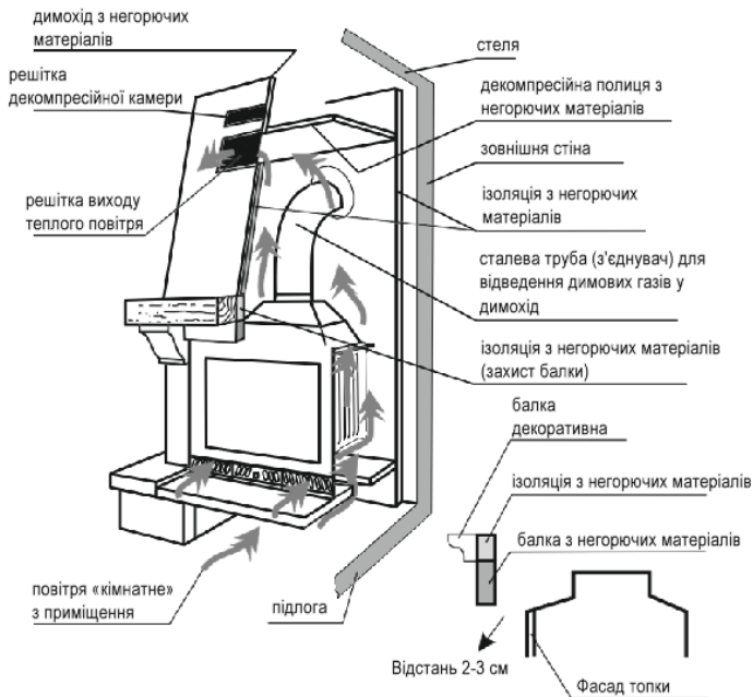
Рис. 2. Приклад способу установки камінної топки
