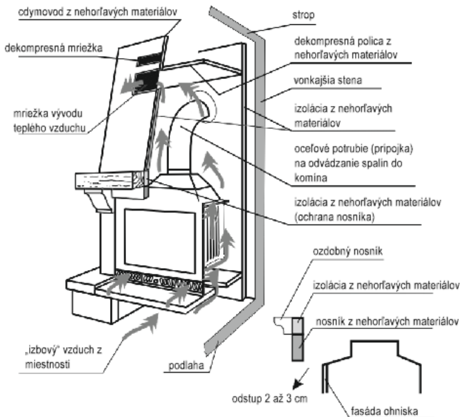
Obr. 2. Názorný spôsob inštalovania krbových vložiek.
