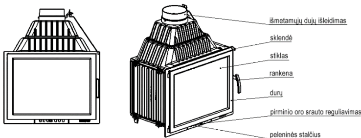
1 pav. Židinio įdėklo schema
