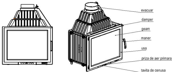
Fig. 1. Schema generala a semineului
