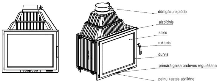
Att. 1 Kamīna ieliktņa shēma.
