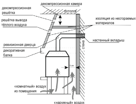
Рис. 3. Примерный способ инсталляции каминных вкладышей - вид сверху и сбоку.
