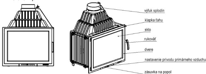
Obr. 1. Schéma krbovej vložky.
