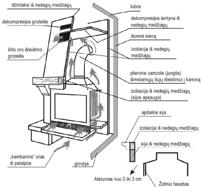
2 pav. Židinio įdėklų įrengimo pavyzdys
