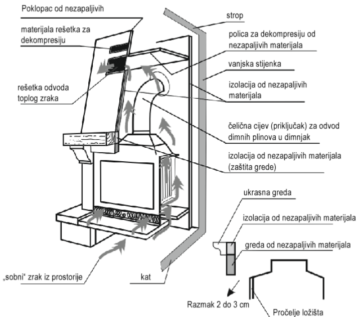
Crtež 2. Primjer načina ugradnje ugradbenih komina
