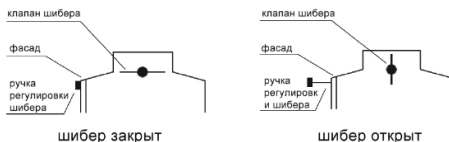
Рис. 5. Примерная регулировка шибер
