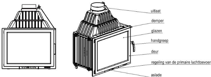
Afb. 1. Schema van de haardpatroon
