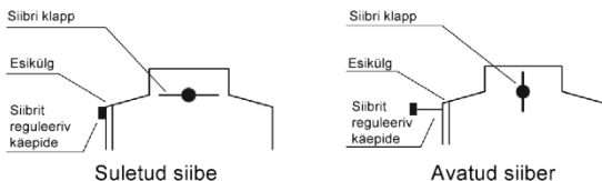
Joonis 5. Näitlik siibri reguleerimine
