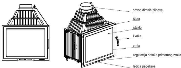
Crtež 1. Shematski prikaz ugradbenog kamina
