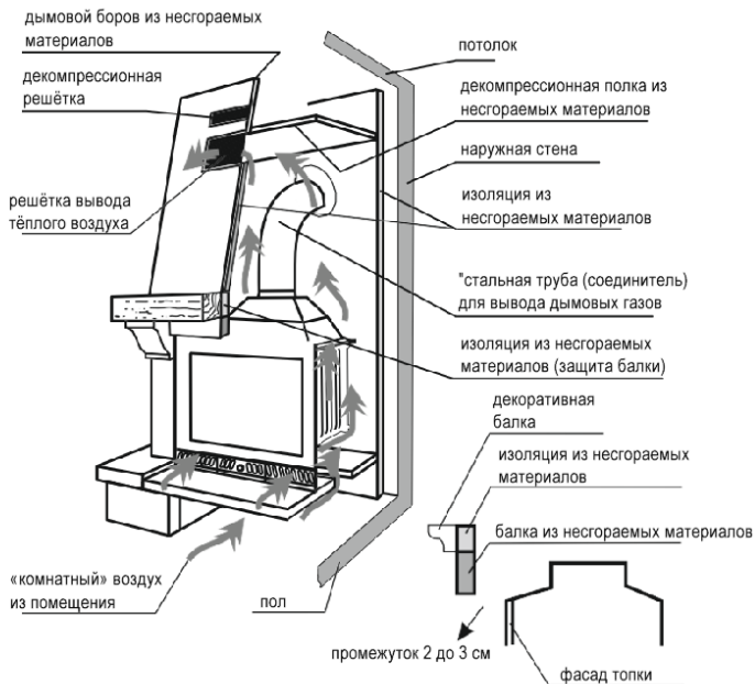
Рис. 2. Примерный способ инсталляции каминных вкладышей.
