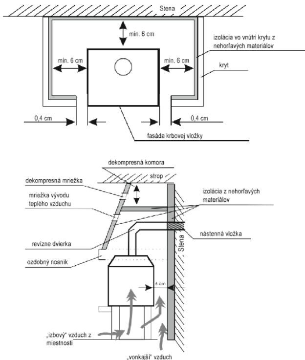
Obr. 3. Názný spôsob inštalovania krbových vložiek - pohľad zhora a z boku.
