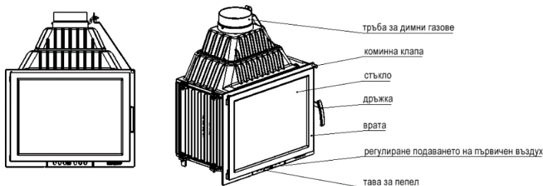
Фиг. 1. Схема на камина за вграждане
