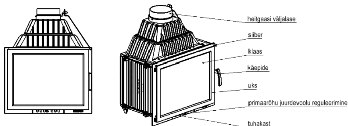
Joonis 1. Kaminasüdamiku skeem
