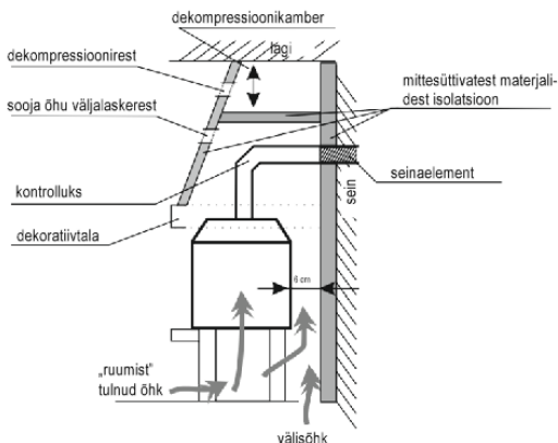
Joonis 3. Näide kaminasüdamike paigaldusest – vaade ülalt ja küljelt
