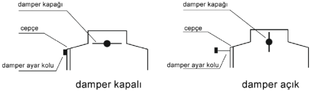
Şek. 4. Havanın hazneye erişiminin ayar örneği (küllük cephesinin görünümü)
