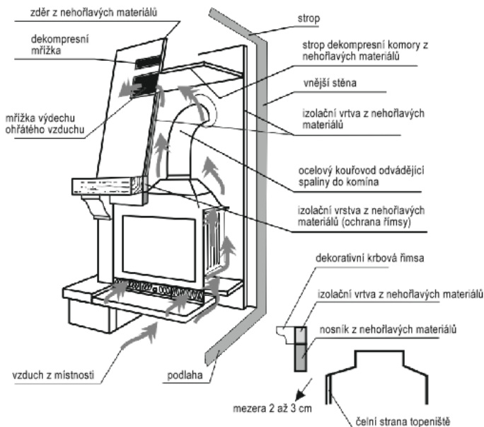
Obr. 2. Příklad montáže krbových vložek.
