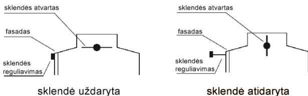
5 pav. Pavyzdinis sklendės reguliavimas
