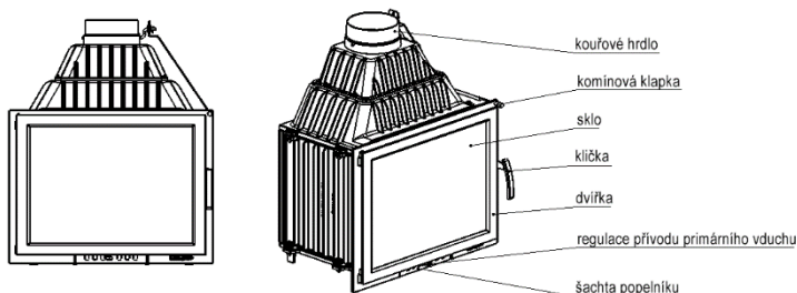
Obr. 1. Schéma krbové vložky
