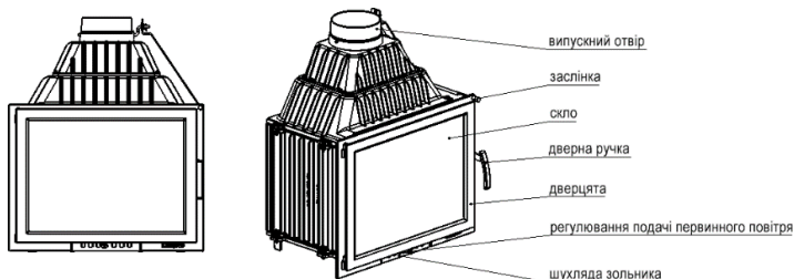
Рис. 1. Схема камінної топки
