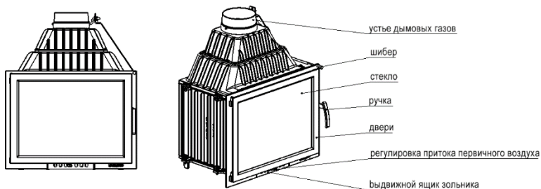
Рис. 1. Схема каминного вкладыша
