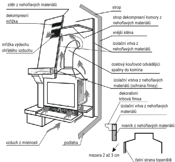
Obr. 2. Příklad montáže krbových vložek.
