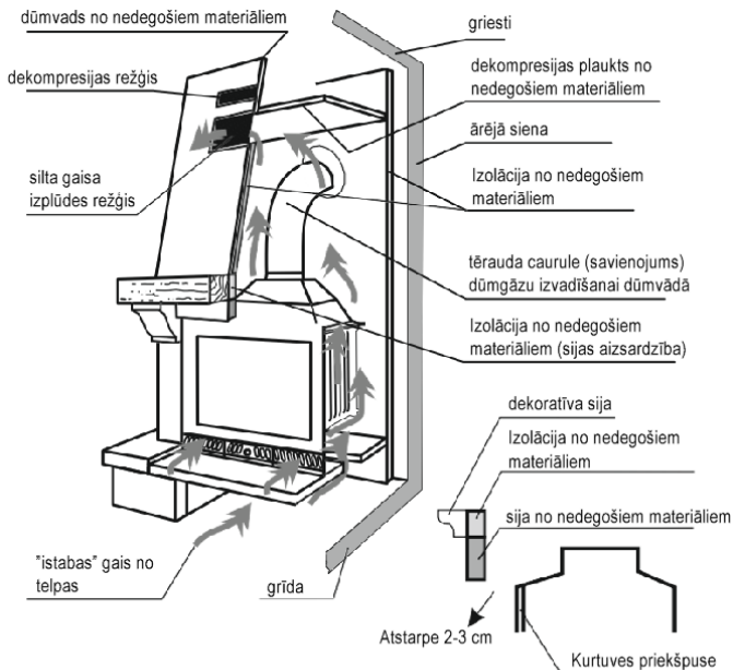
Att. 2 Piemērs, kā uzstādīt kamīna ieliktnus.
