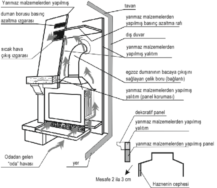
Şek. 2. Şömine haznelerinin kurulum şekli örneği
