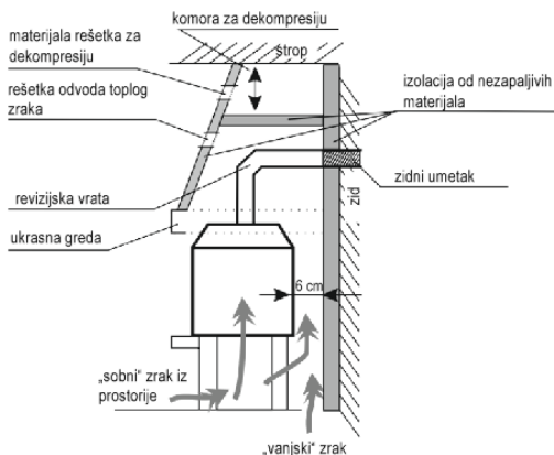
Crtež 3. Primjer načina ugradnje ugradbenih komina - tlocrt i bokocrt
