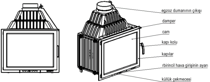
Şek. 1. Şömine haznesi şeması
