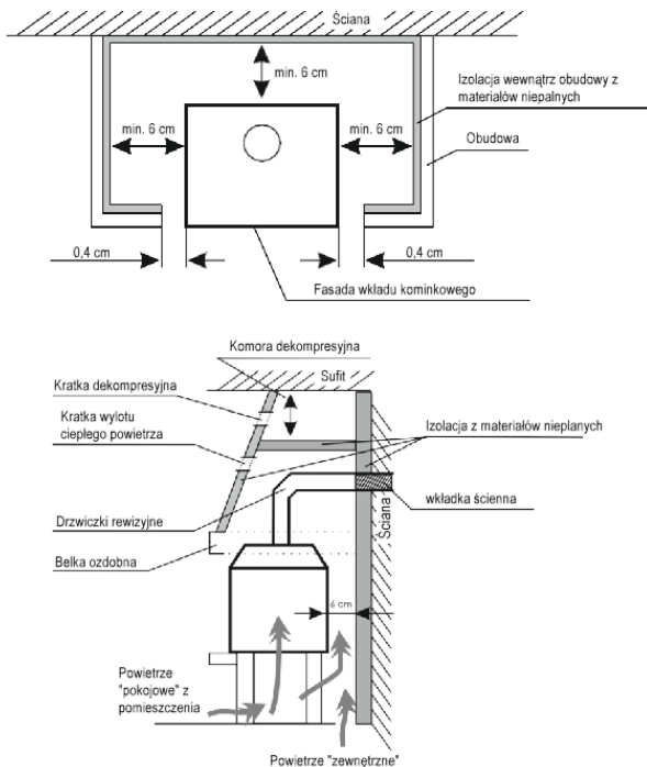
Rys. 3. Przykładowy sposób instalacji wkładów kominkowych - widok z góry i z boku
