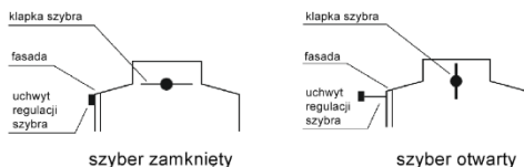
Rys. 5. Przykładowa regulacja szybra.
