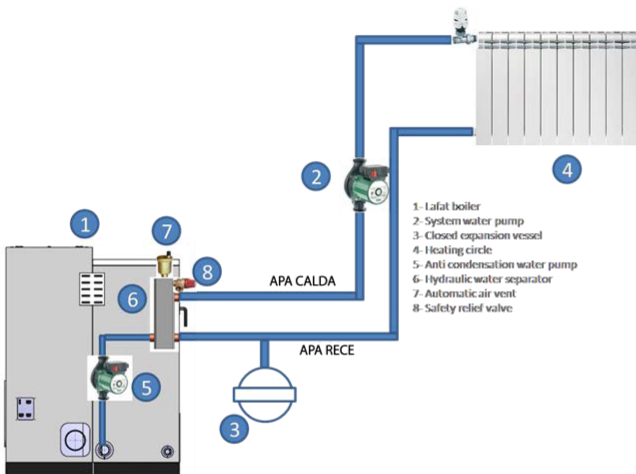
Figura 23. Schema instalației hidraulice
