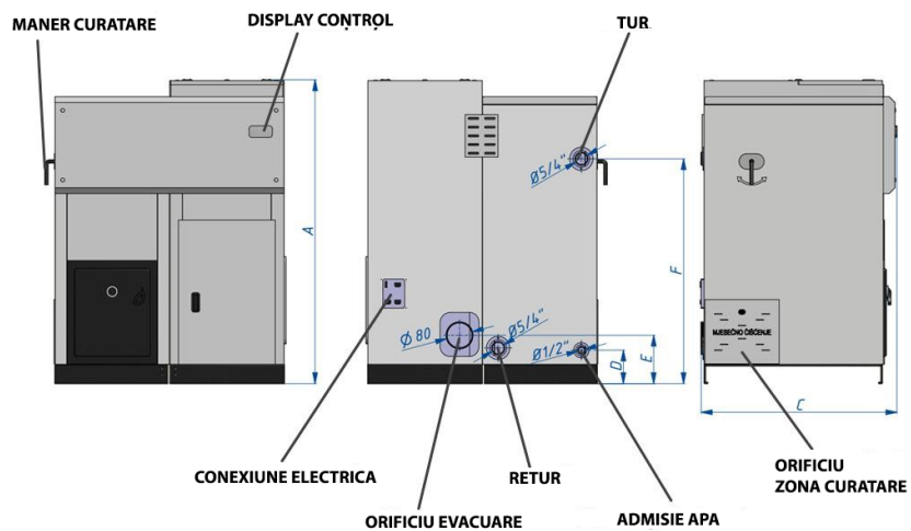
Figura 1. Centrală SM ECO 35-100 (kW)
