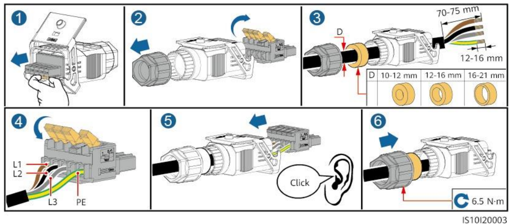
Figura 5-6 Cablu cu patru conductori (L1, L2, L3 și PE)
