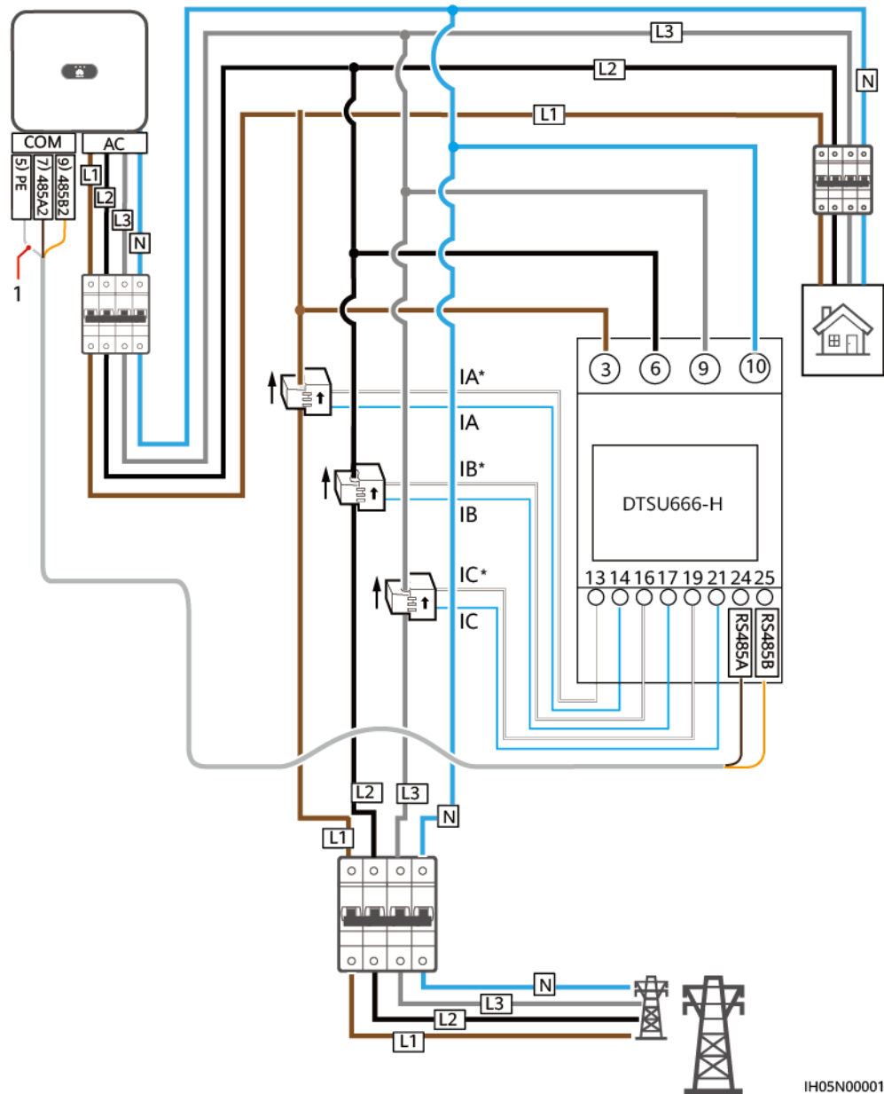
Figura 5-24 Conexiune cablu (cablu trifazat cu patru conductori)
