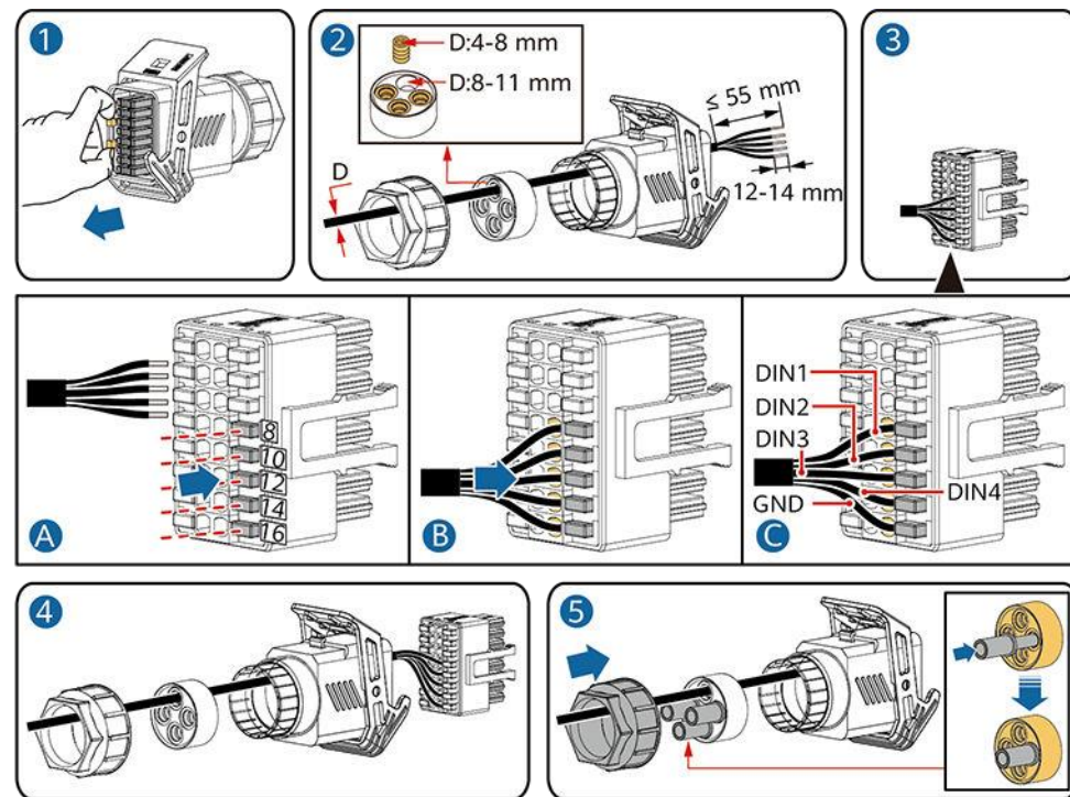
Figura 5-30 Instalarea cablului
