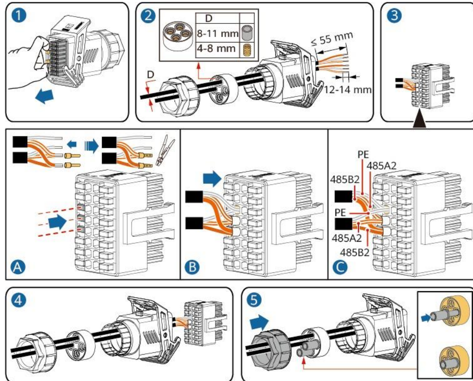
Figura 5-27 Instalarea cablului
