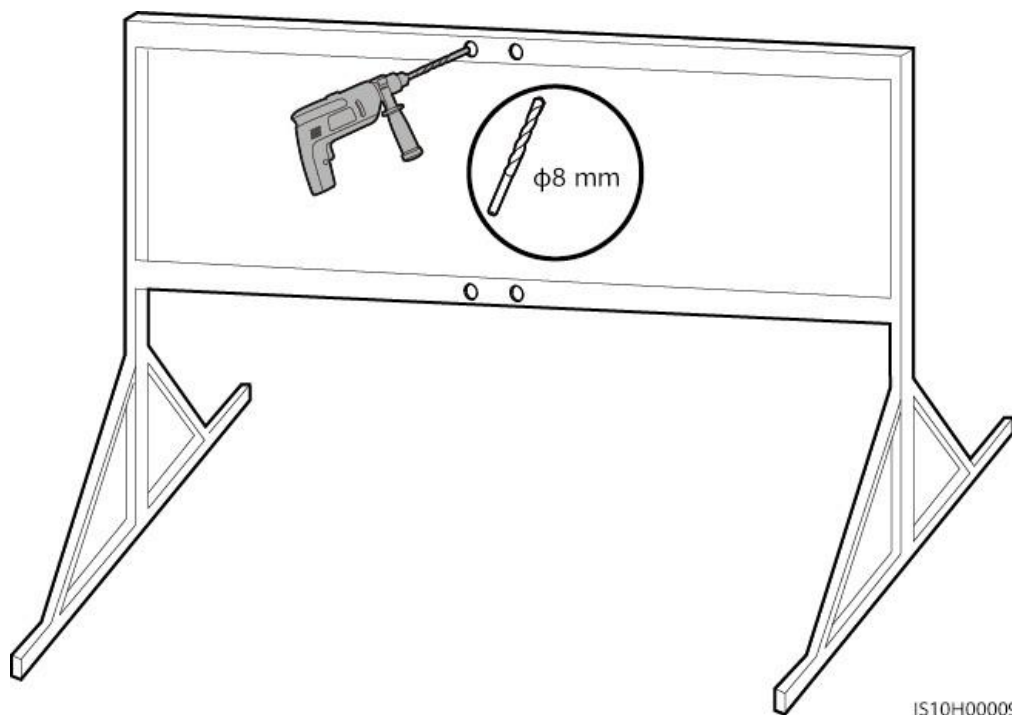
Figura 4-14 Executarea găurilor
