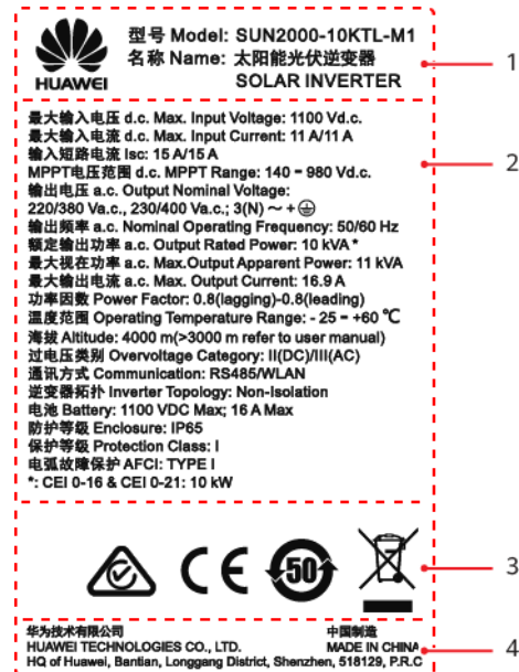
Figura 2-5 Plăcuță de identificare (folosind ca exemplu SUN2000-10KTL-M1)
