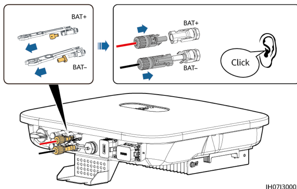
Figura 5-15 Conectarea cablurilor bateriei
