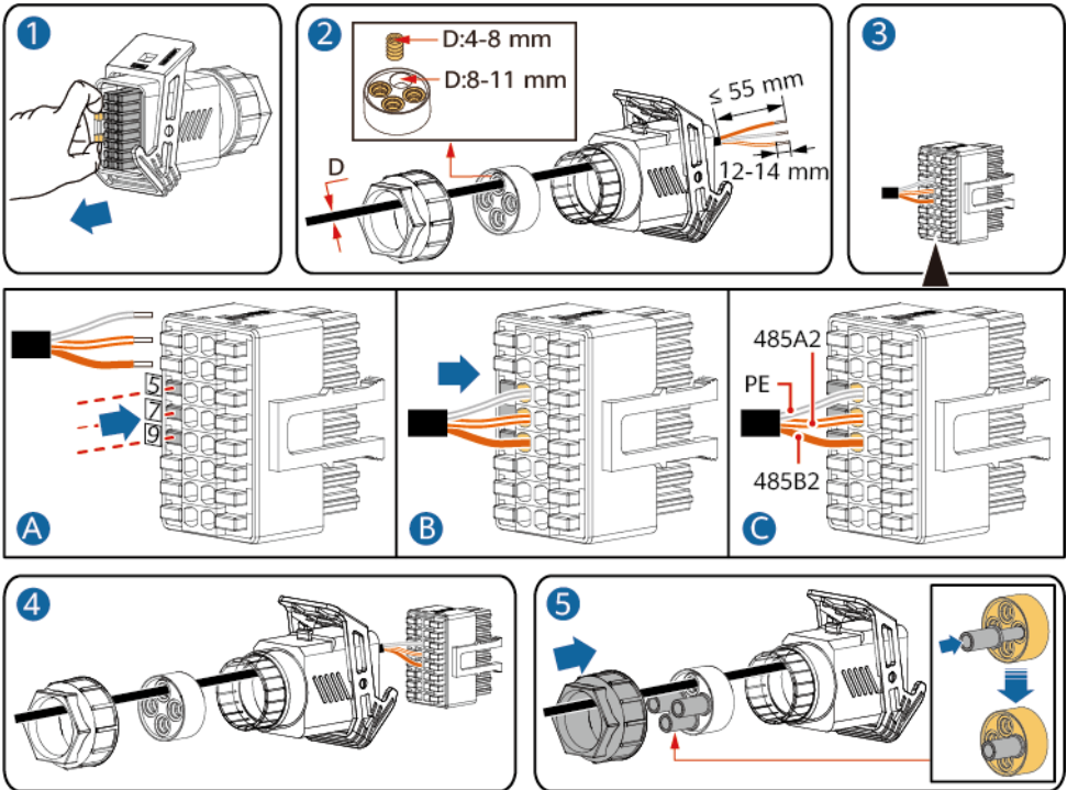
Figura 5-25 Instalarea cablului
