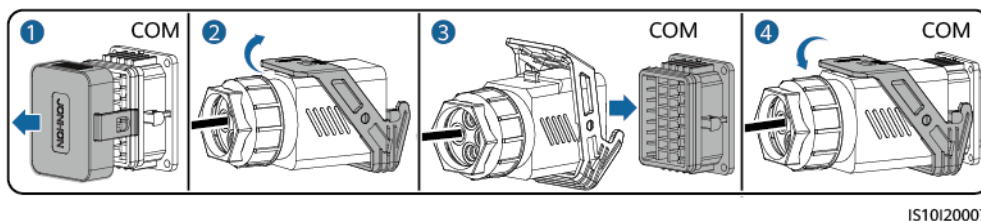
Figura 5-31 Fixarea conectorului cablului de
