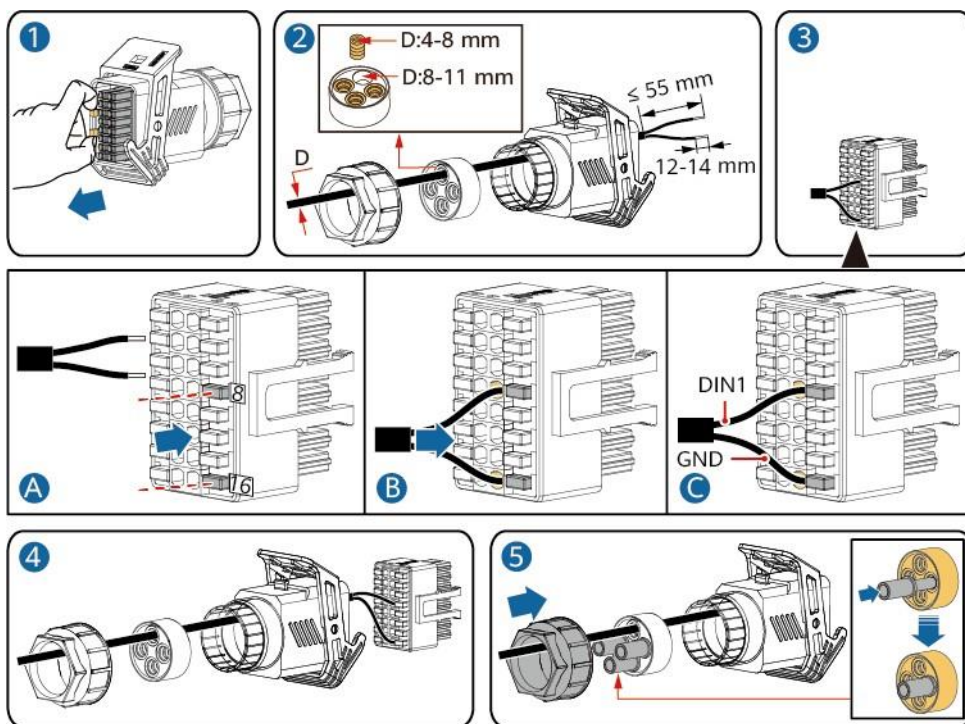
Figura 5-32 Instalarea cablului
