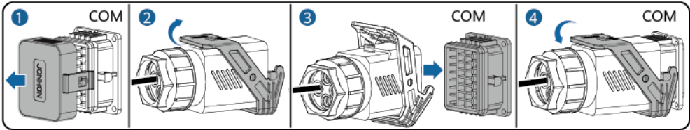
Figura 5-33 Fixarea conectorului cablului de
