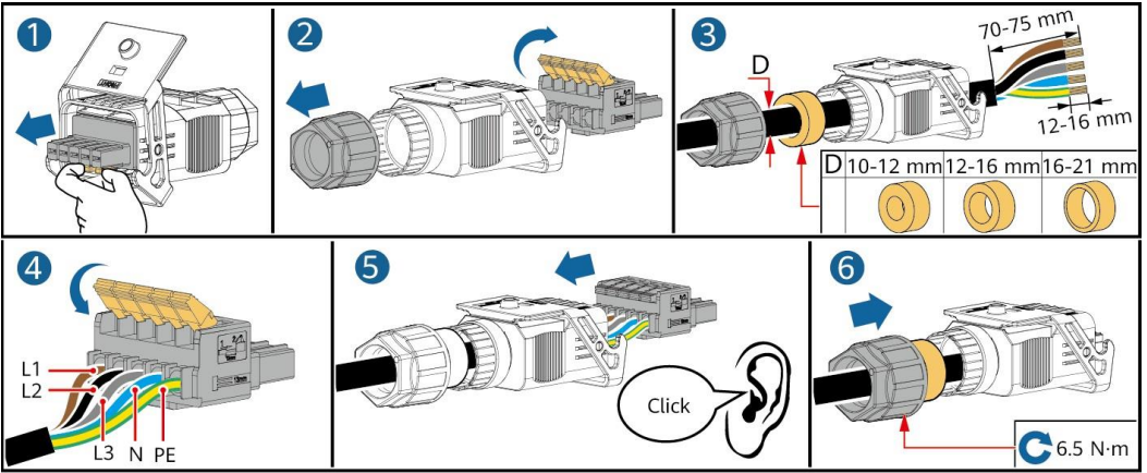
Figura 5-8 Cablu cu cinci conductori (L1, L2, L3, N și PE)
