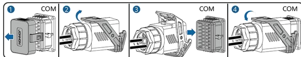
Figura 5-28 Fixarea conectorului cablului de semnal
