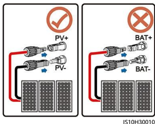
Figura 5-12 Borne de cablare corecte
