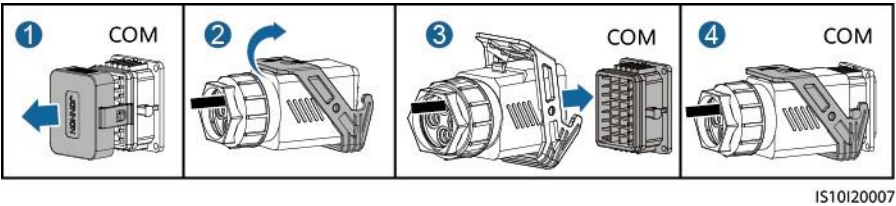
Figura 5-26 Fixarea conectorului cablului de semnal
