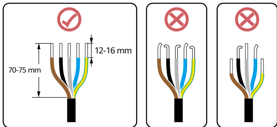
Figura 5-5 Cerințe de sertizare
