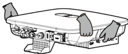
Figura 4-6 Mutarea SUN2000
