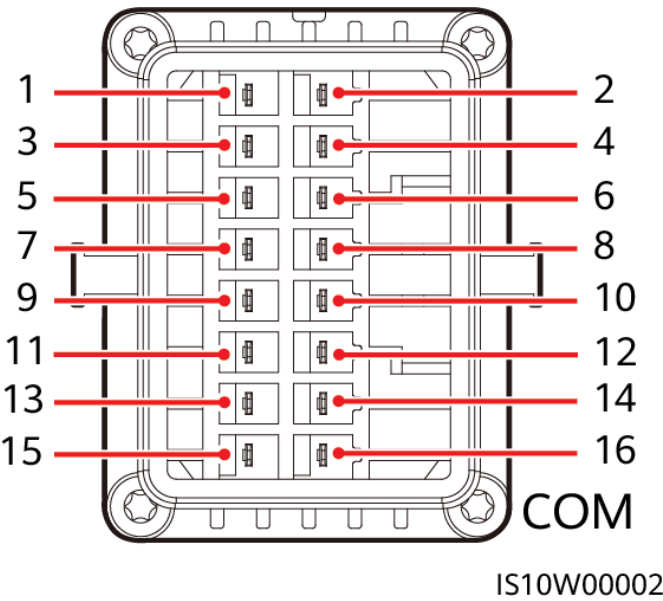
Figura 5-18 Definiții pini
