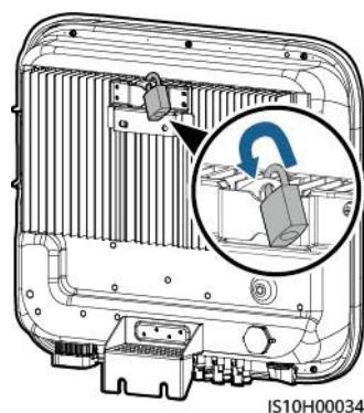
Figura 4-18 Instalarea încuietorii antifurt
