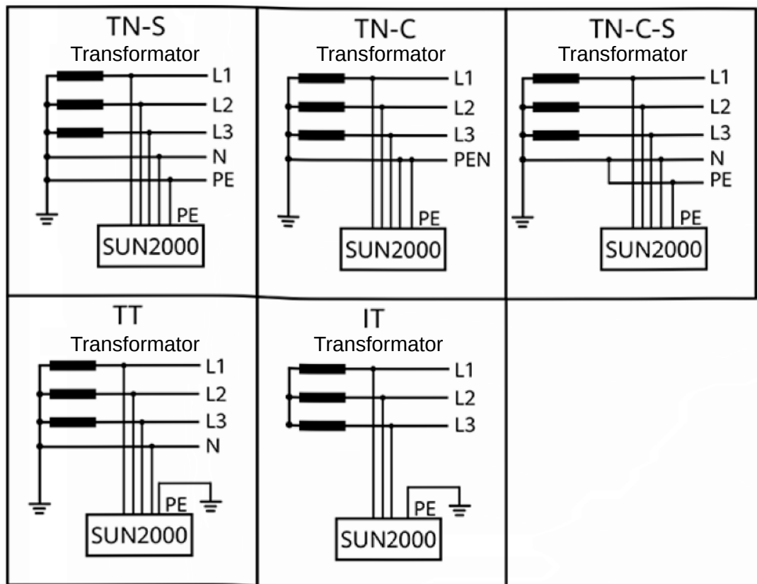
Figura 2-6 Rețele electrice acceptate
