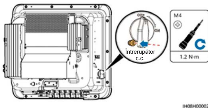
Figura 4-8 Instalarea șurubului de blocare a întrerupătorului c.c.
