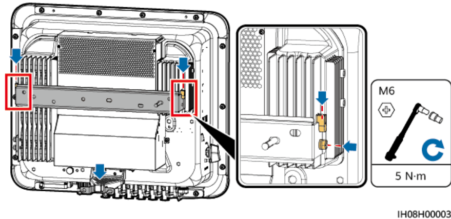
Figura 4-9 Instalarea invertorului
