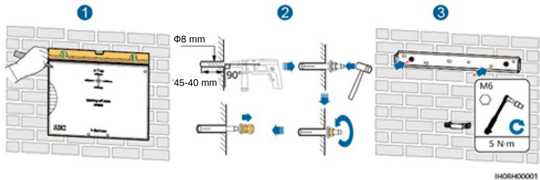
Figura 4-7 Instalarea suportului de montare
