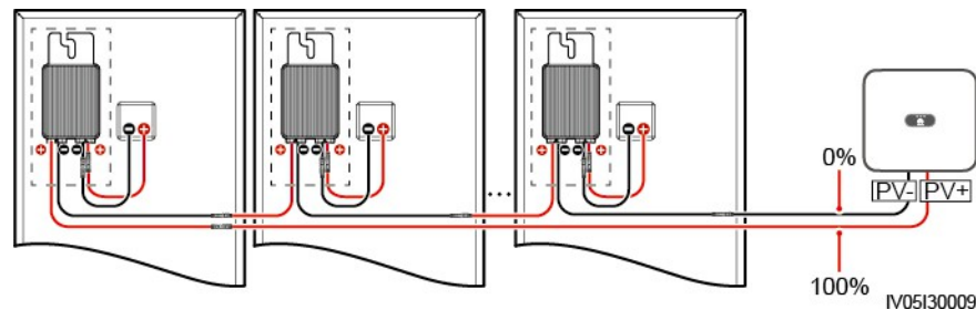
Figura 8-2 Procentul pozițiilor de scurtcircuit
