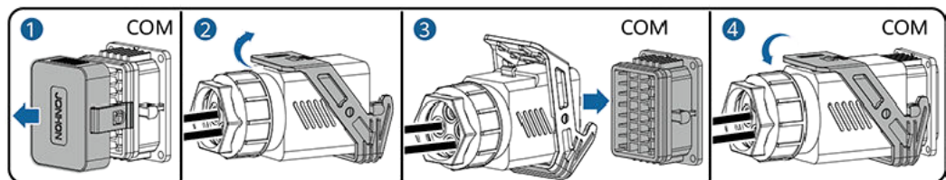
Figura 5-21 Fixarea conectorului cablului de semnal
