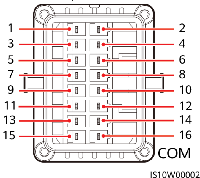
Figura 5-16 Definiții pini
