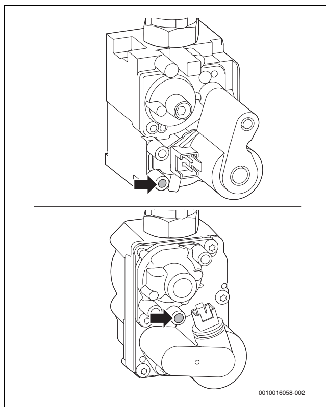
Fig. 48 Orificiu de măsurare pentru presiunea de racordare a gazului
