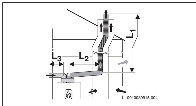
Fig. 13 Flexible Abgasführung nach C_{53} im Schacht und getrennte einwandige Luftzufuhr- und Abgas-Leitungen im Aufstellraum
