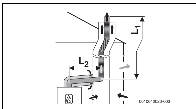
Fig. 17 Flexible Abgasführung im Schacht nach B 53p mit raumluftabhängiger Luftzufuhr über die konzentrische Verbindungsleitung im Aufstellraum; Hinterlüftungsöffnung im Schacht
