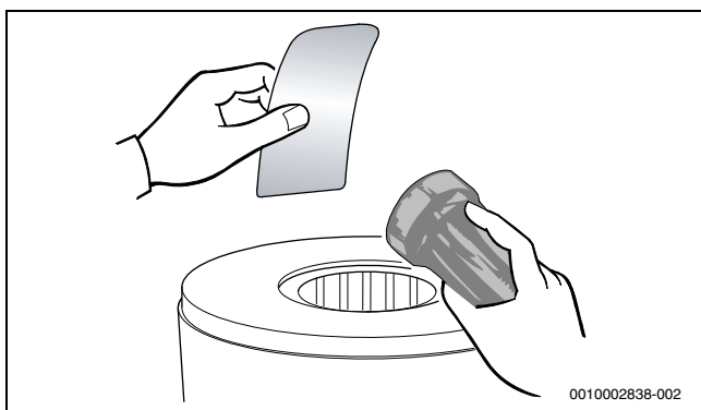
Fig. 58 Verificarea blocului de căldură în privința reziduurilor
