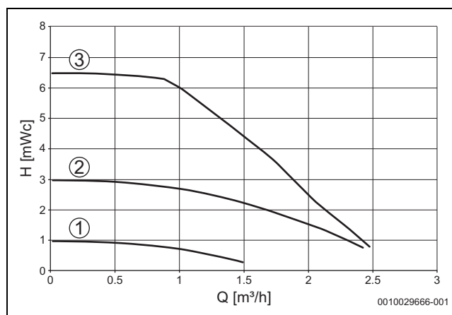
Fig. 44 Curbă caracteristică a pompei pentru circuitul de încălzire (presiune constantă)
