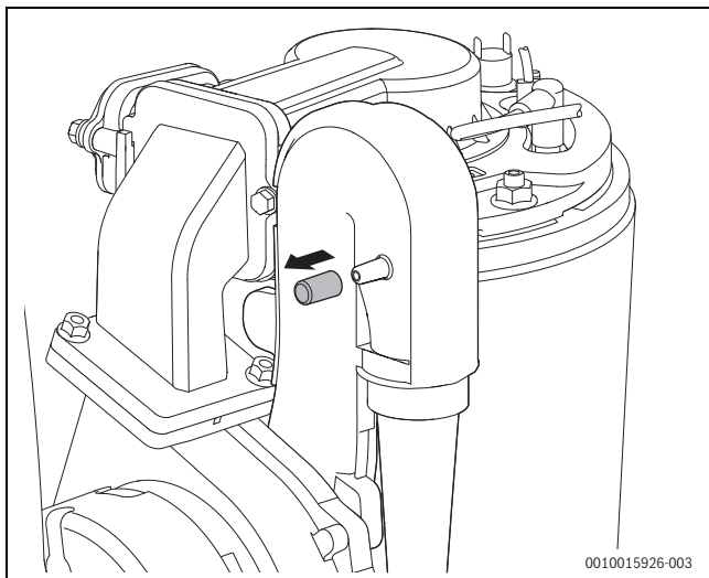
Fig. 50 Orificiu de măsurare al sistemului de amestecare
