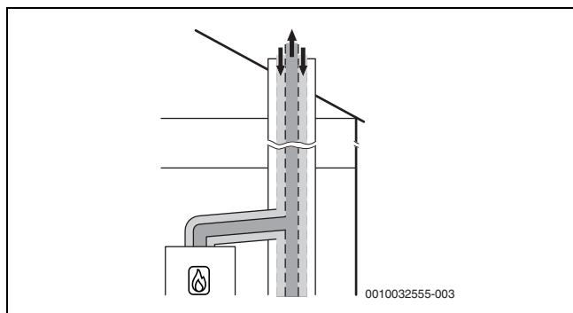
Fig. 10 Ghidarea concentrică a aerului/gazelor arse conform C 43x în încălăperea centralei termice
