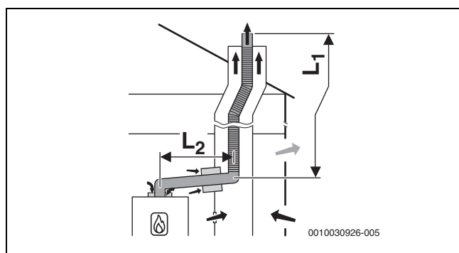
Fig. 19 Flexible Abgasführung im Schacht nach B 53P mit raumluftabhängiger Luftzufuhr am Gerät und einwandiger Abgasleitung im Aufstellraum; Hinterlüftungsöffnung im Schacht
