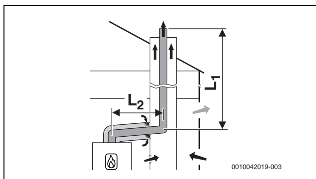
Fig. 16 Ghidarea rigidă a gazelor arse în puț conform B 53p cu alimentare cu aer dependentă de aerul din încălăt prin tronsonul de legătură concentric în încăperea centralei termice; aerisire posterioară în puț
