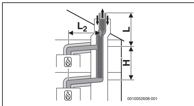
Fig. 26 Mehrfachbelegung nach C (14)3x mit kollektiver flexibler Abgasführung und konzentrischer Luft-Abgas-Führung im Aufstellraum
