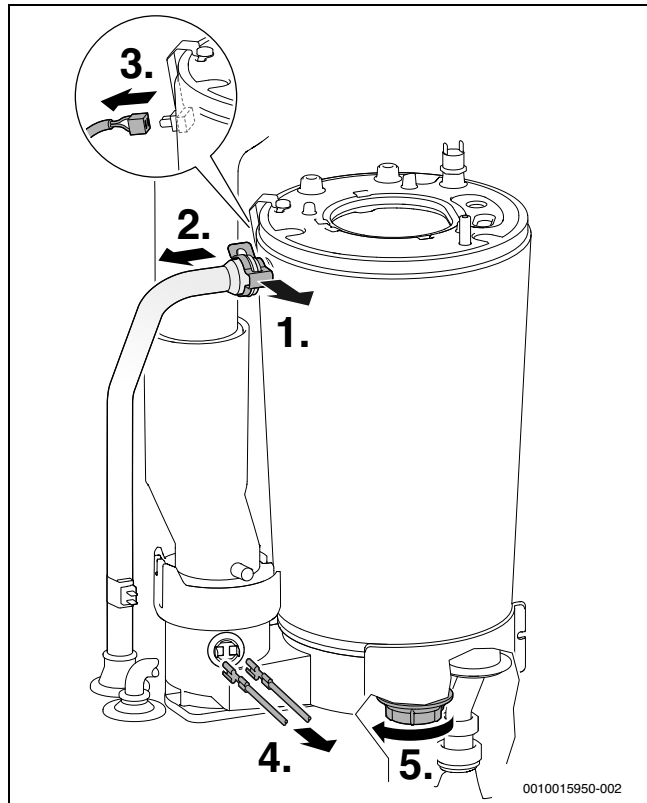
Fig. 74 Desprinderea țevii de tur și scoaterea cablului
