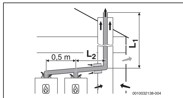
Fig. 27 Cascadă cu 2 aparate: Ghidarea rigidă a gazelor arse în puț conform B 53p cu alimentare cu aer dependentă de aerul din încăpă la nivelul aparatului și tubulatură pentru gaze arse cu un perete în încăperea centralei termice; aerisire posterioară în puț
