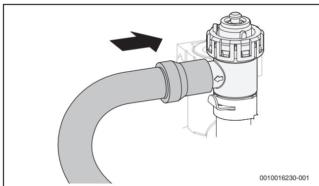
Fig. 33 Montarea furtunului la supapa de siguranță
