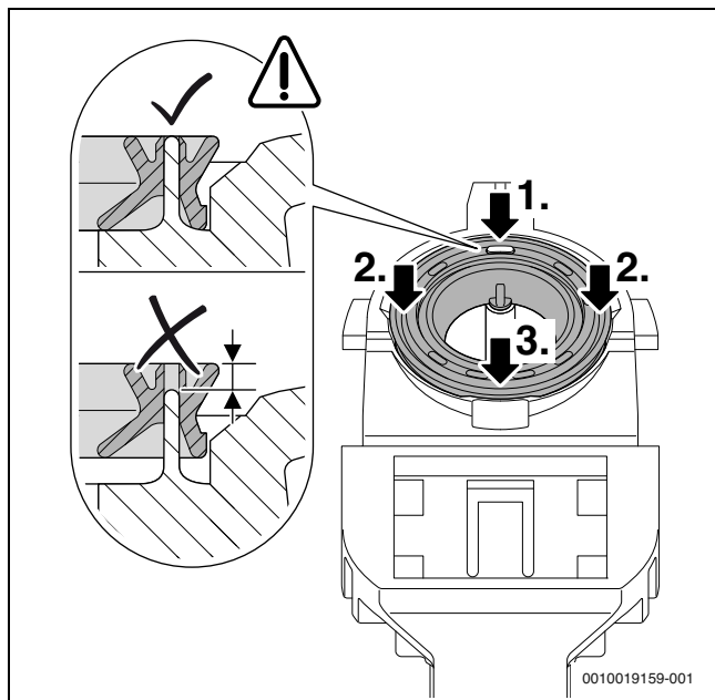
Fig. 64 Fixarea prin apăsare a garniturii de etanșare
