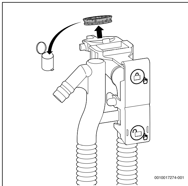
Fig. 62 Îndepărtarea garniturii de etanșare de pe partea superioară a sifonului pentru condensat
