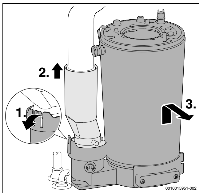
Fig. 75 Demontarea schimbătorului de căldură
