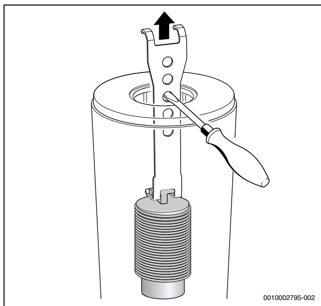
Fig. 56 Scoaterea corpului de întrepătrundere inferior
