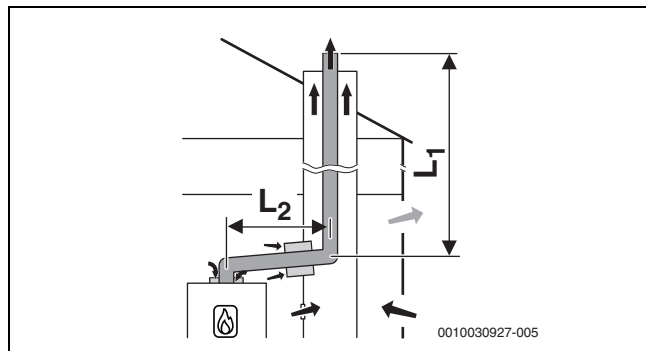
Fig. 18 Ghidarea rigidă a gazelor arse în puț conform B 53P cu alimentare cu aer dependentă de aerul din încălț la nivelul aparatului și tubulatură pentru gaze arse cu un perete în încăperea centralei termice; aerisire posterioară în puț
