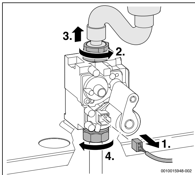
Fig. 69 Scoaterea ștecărului și desfacerea piulițelor oarbe
