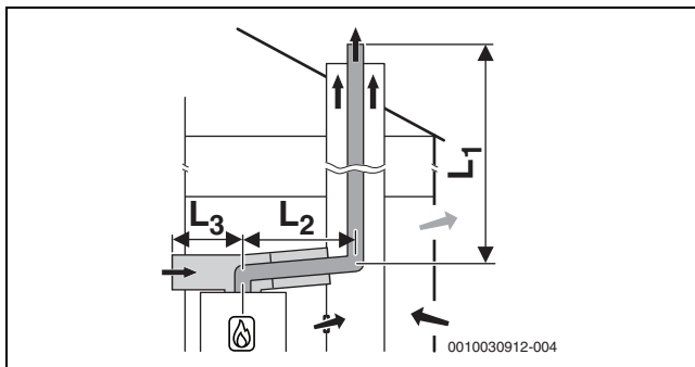
Fig. 11 Ghidarea rigidă a gazelor arse în puț conform C 53x și ghidarea aerului/gazelor arse cu alimentare cu aer separată și evacuare concentrică a gazelor arse în încălăperea centralei termice
