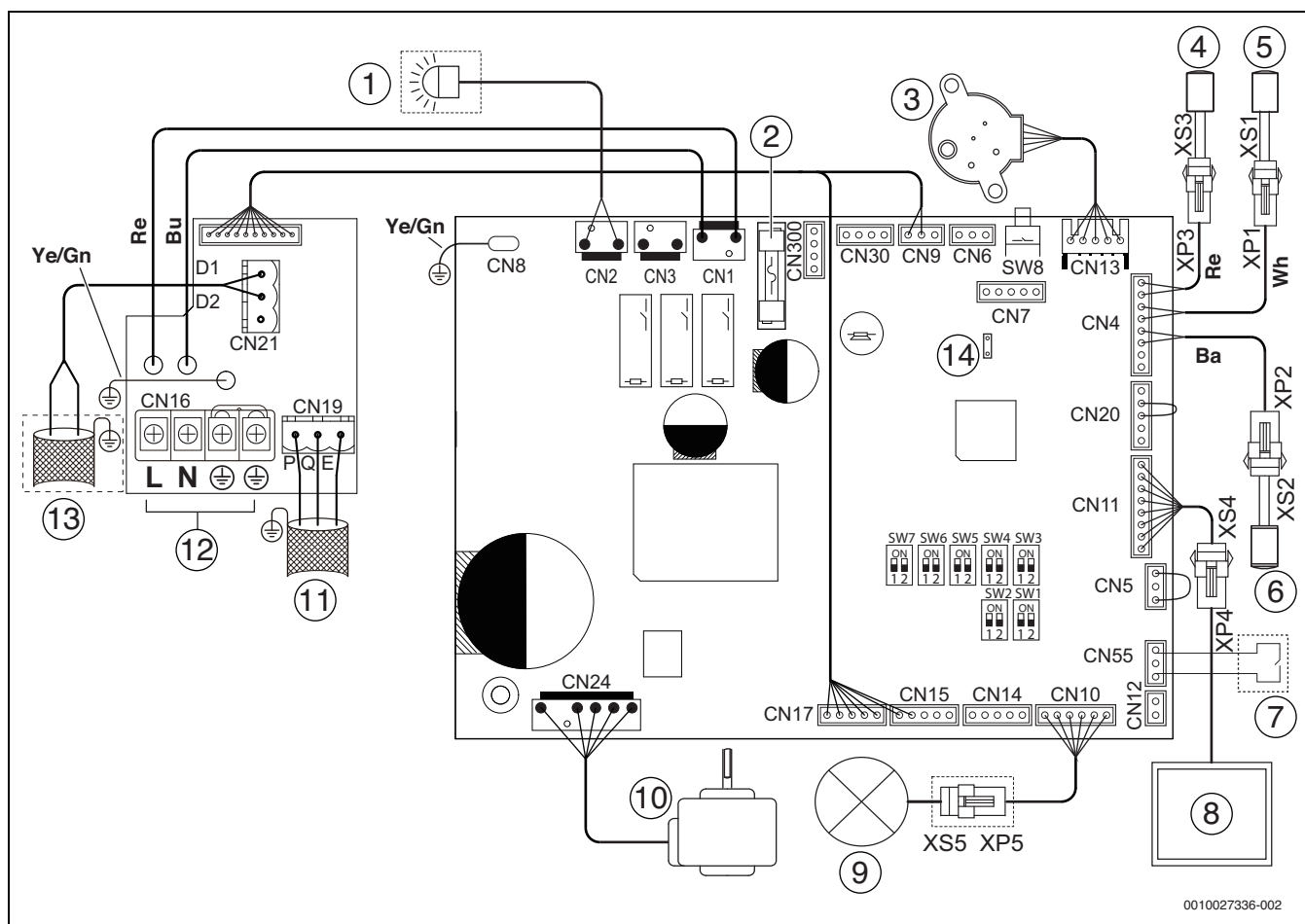
Fig. 34 Cablarea electrică, model 17
