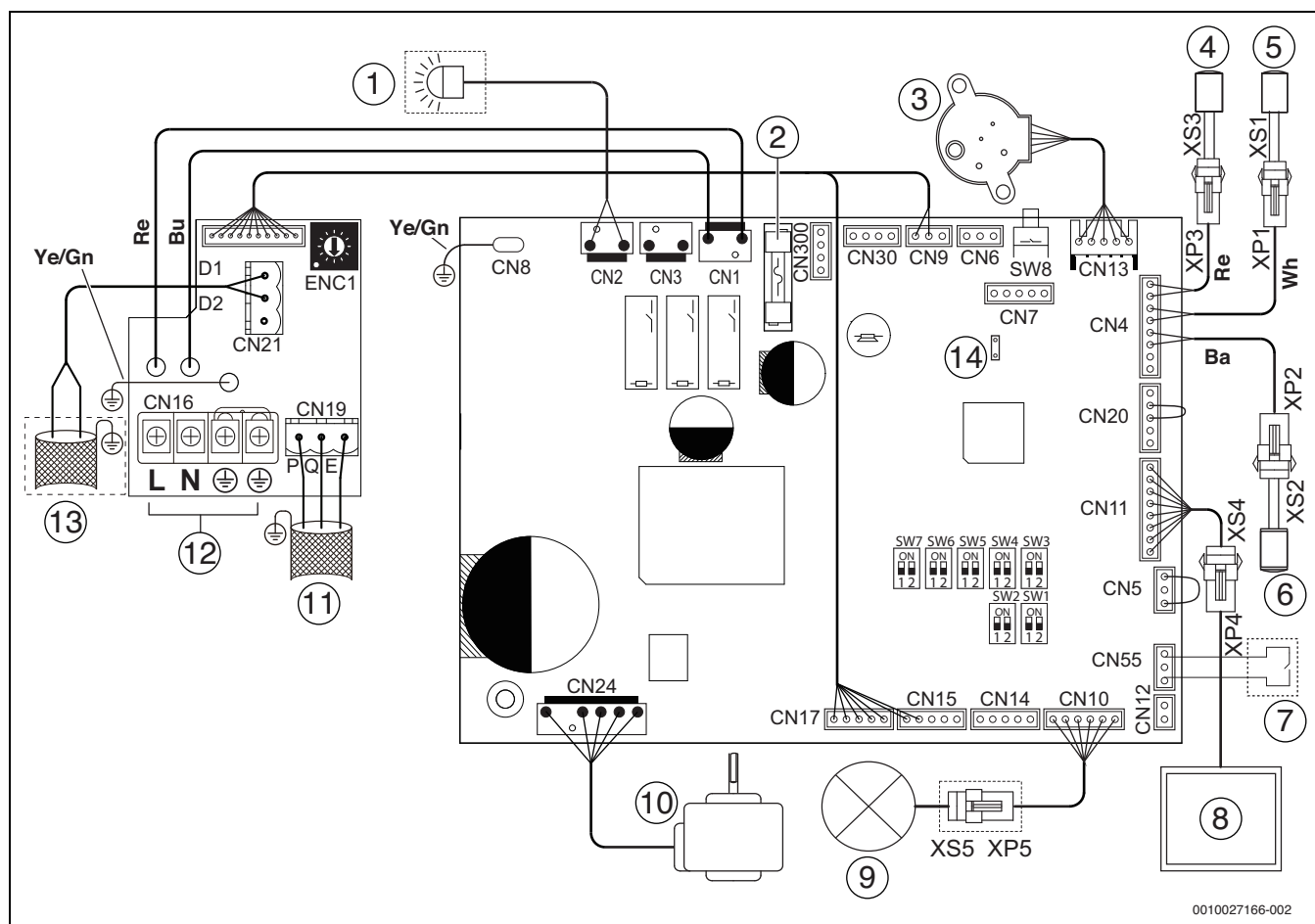
Fig. 35 Cablare electrică, modelele 22 - 28
