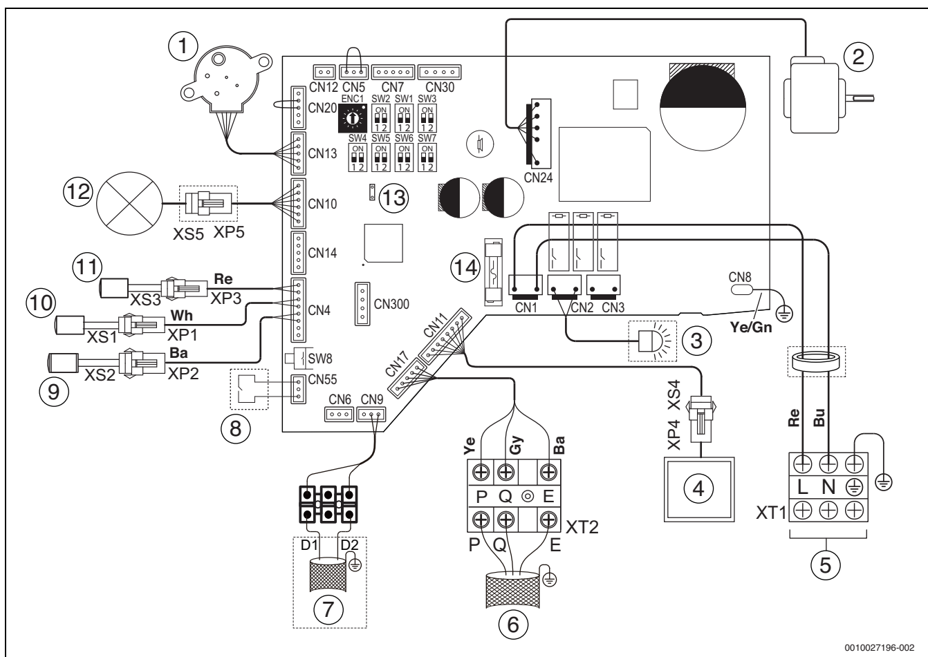
Fig. 36 Cablare electrică, modelele 36 - 56
