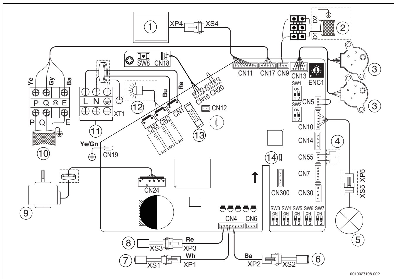
Fig. 37 Cablare electrică, modelele 71 - 90
