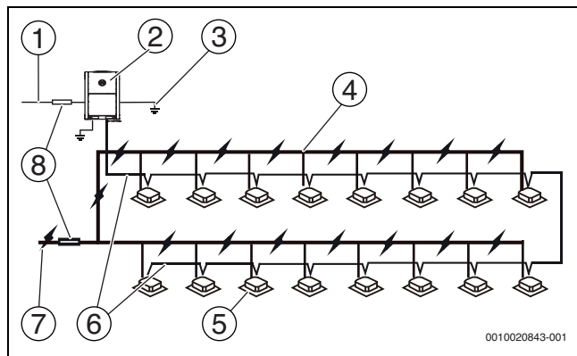
Fig. 19 Terminalul de alimentare cu energie electrică al unității interioare
