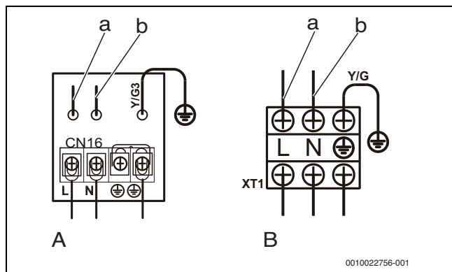
Fig. 20 Terminalul de alimentare cu energie electrică al unității interioare.
