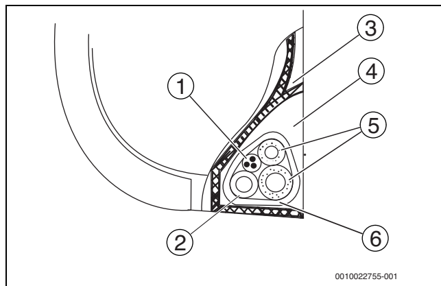
Fig. 15 Vedere laterală a unității interioare
