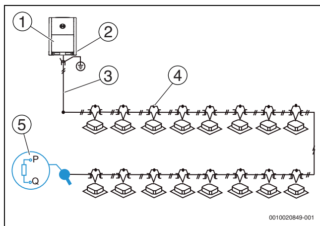
Fig. 39 Cablu de comunicare între unitățile interioare și unitatea exterioară (PQE)
