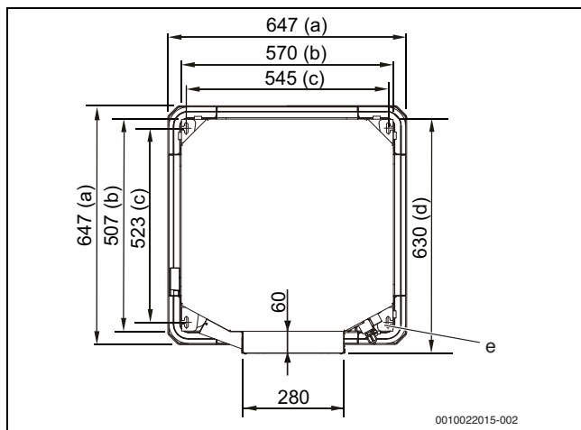
Fig. 14 Dimensiunile unității [mm]
