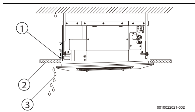
Fig. 20 Scurgeri de aer și apă
