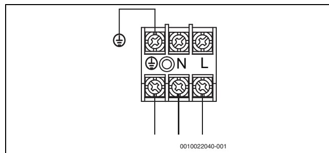
Fig. 35 Alimentarea cu energie
