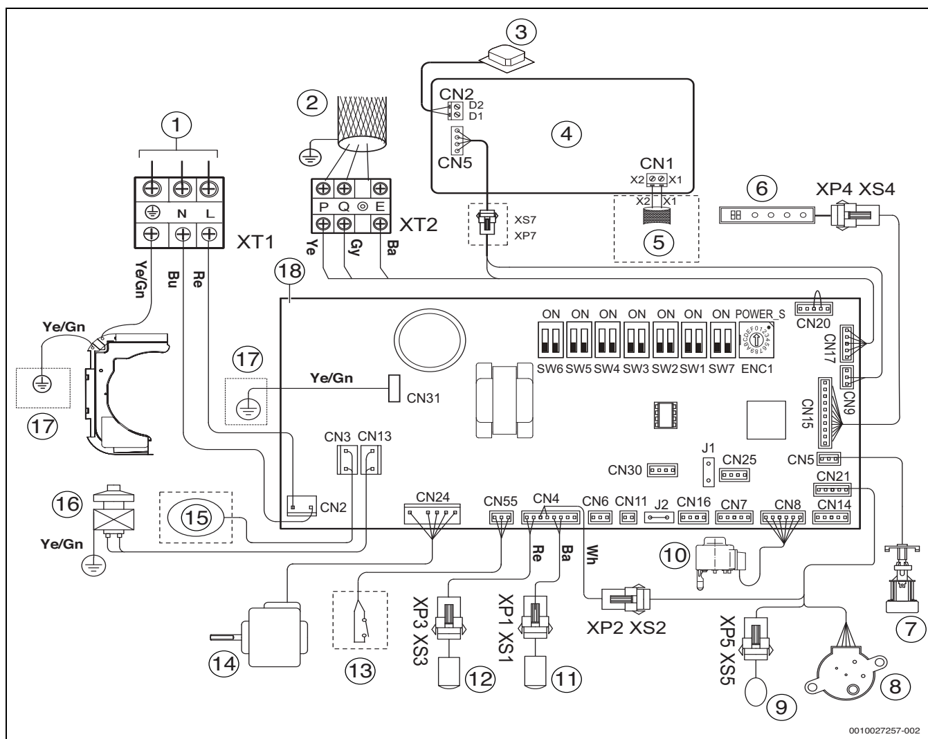
Fig. 51 Cablarea electrică
