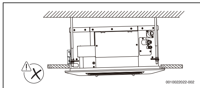
Fig. 21 Nu este permisă existența spațiilor goale
