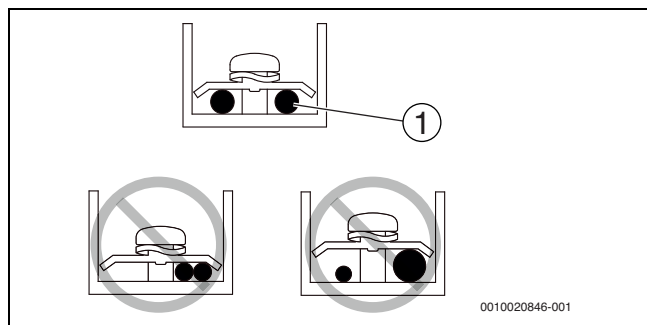
Fig. 37 Conexiuni de cablare corespunzătoare și necorespunzătoare
