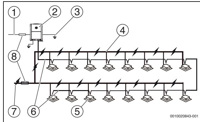
Fig. 34 Terminalul de alimentare cu energie electrică al unității interioare
