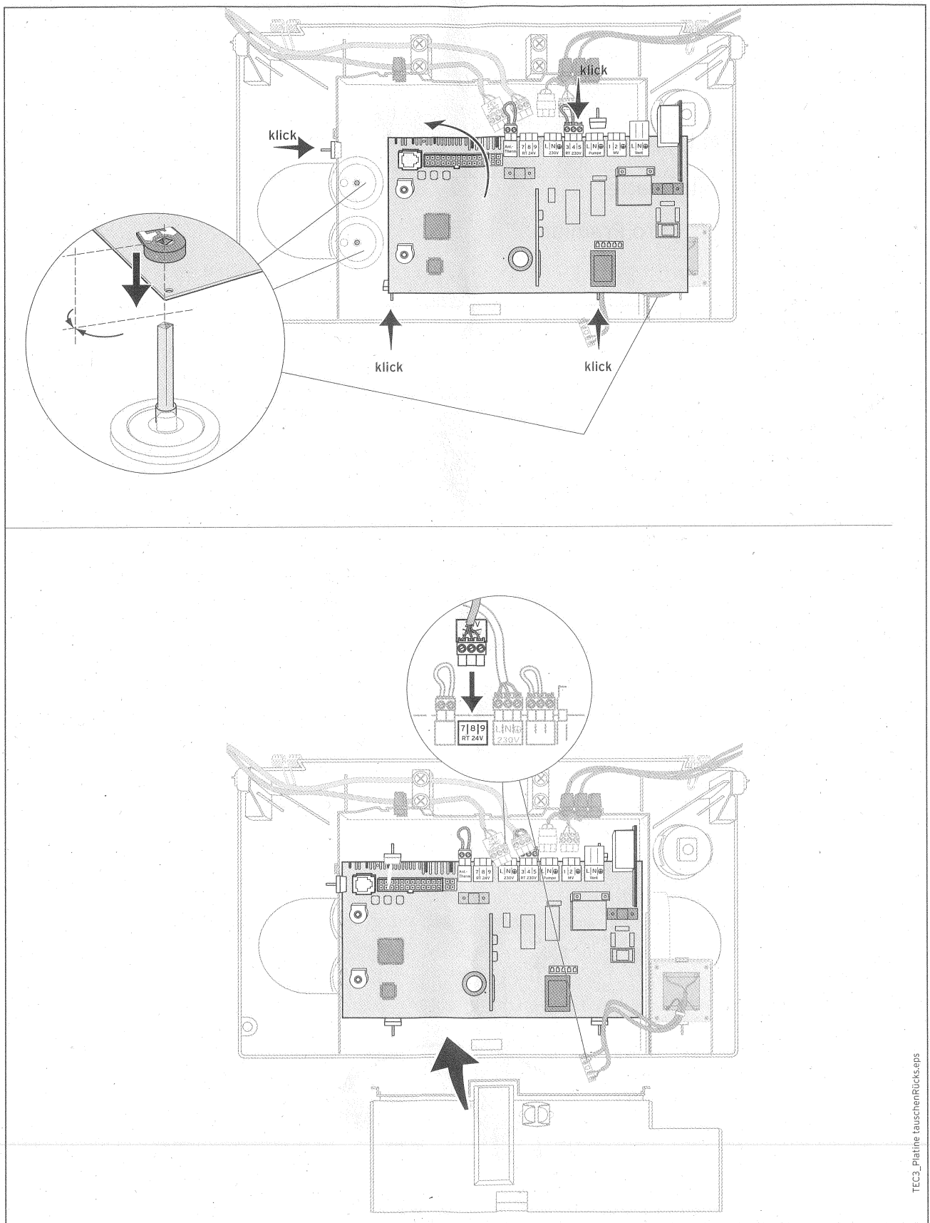
Abb. 2: Platine einbauen
