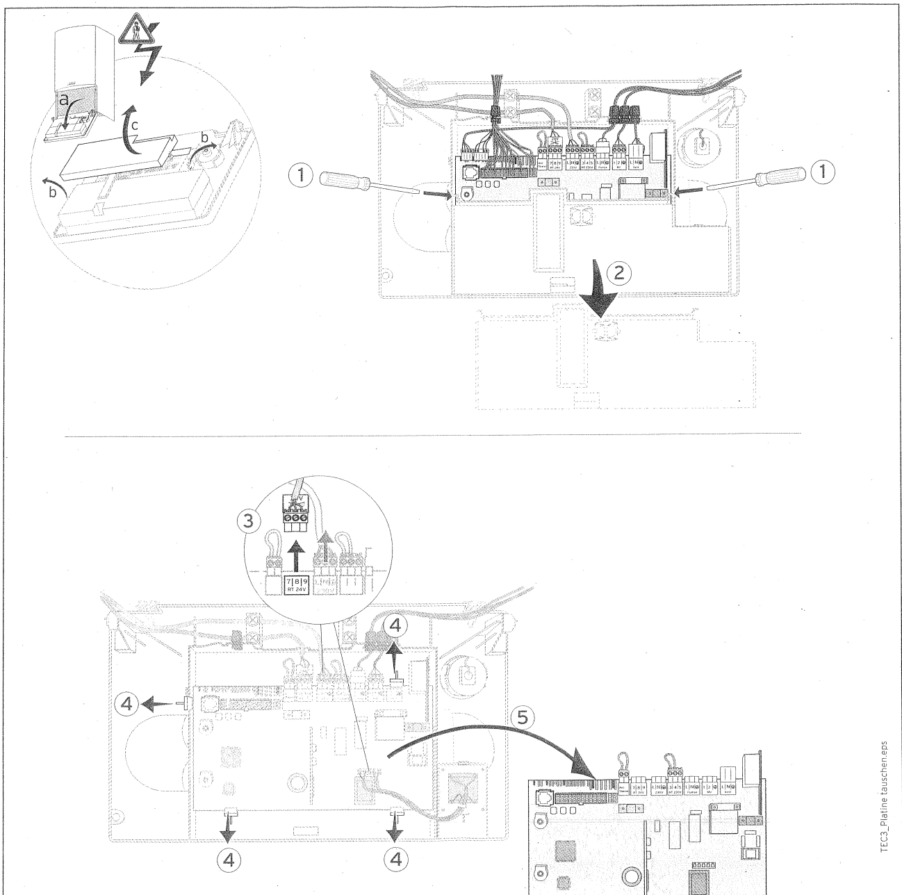
Abb. 1: Platine ausbauen
