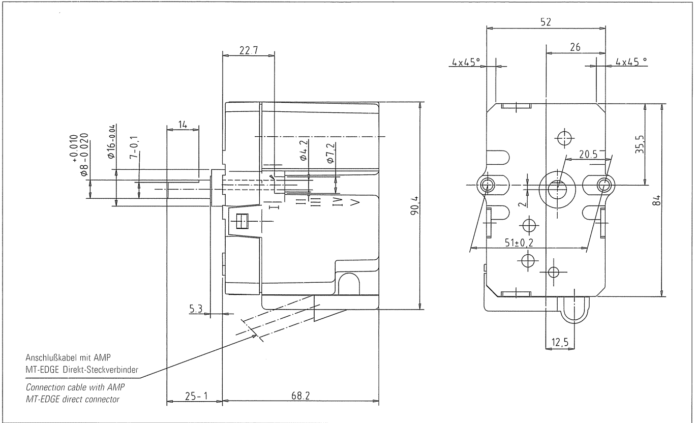
Stellantrieb mit runder Welle / Actuator with round shaft
