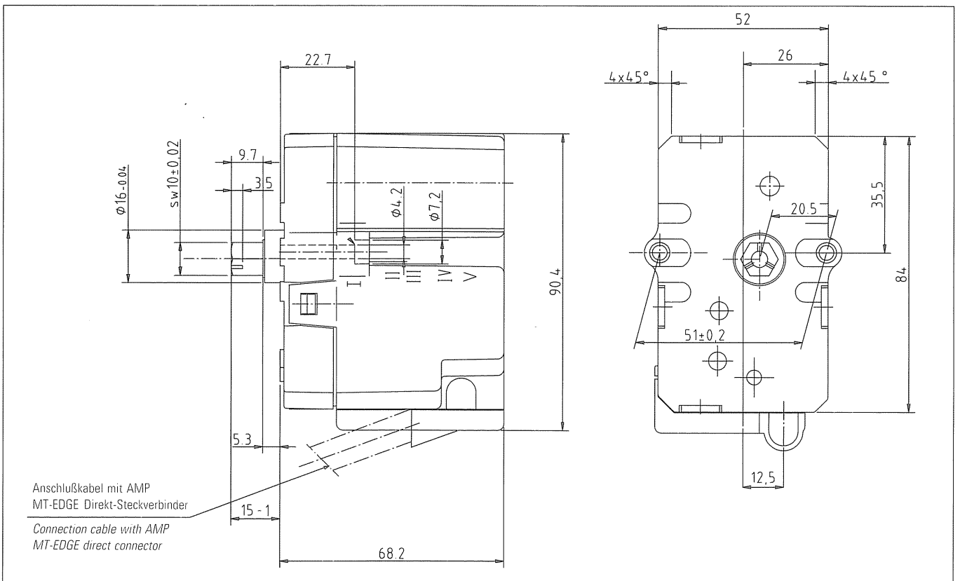
Stellantrieb mit Sechskant-Welle / Actuator with hexagon shaft
