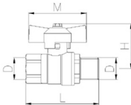
art 434R Robinet cu sfera gaz trecere totala MF , cu maneta fluture
