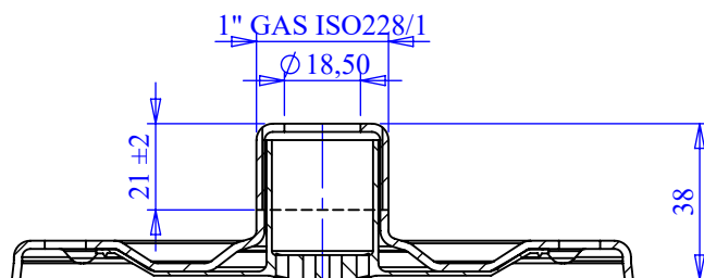
SEZIONE A-A
