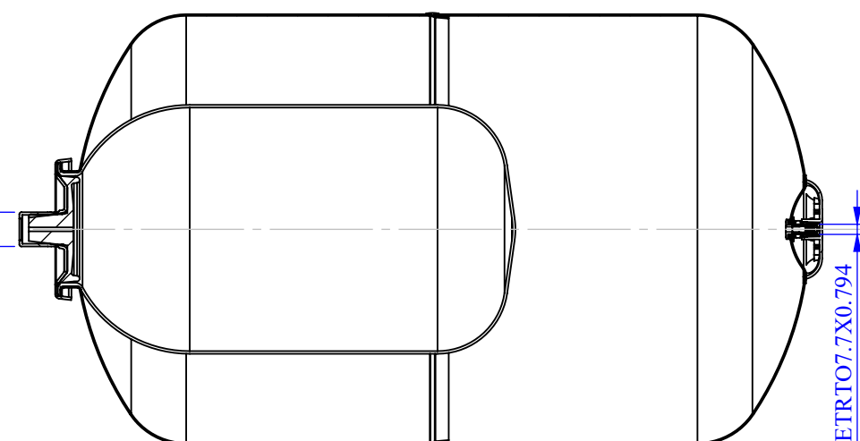
SEZIONE A-A
