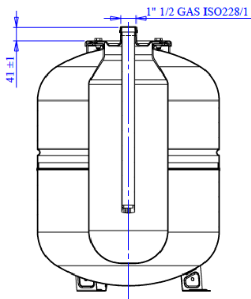
SECTIUNE M-M
