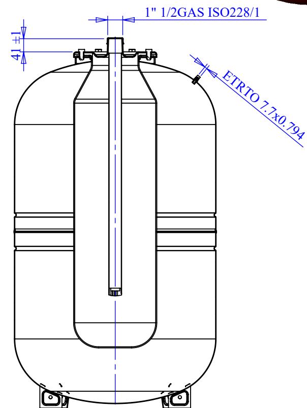
SEZIONE A-A
