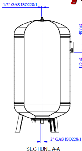
SECTIUNE A-A
