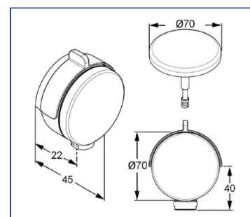
Schiță tehnică
