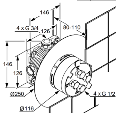
Schiță tehnică
