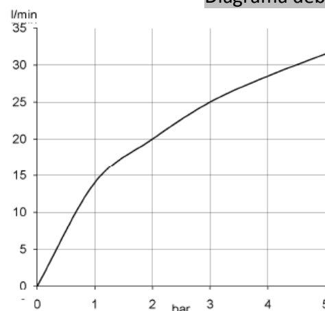
Diagramă debit
