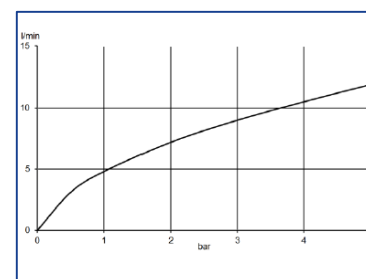
Diagramă debit
