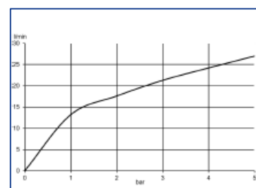
Diagramă de debit
