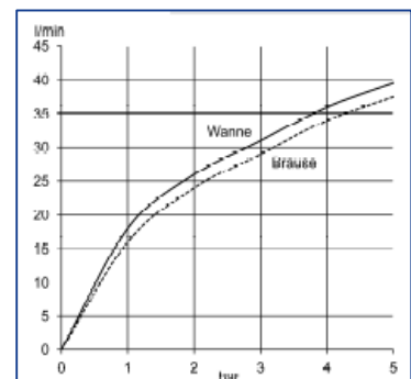
Diagramă debit
