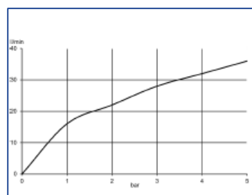
Diagramă debit
