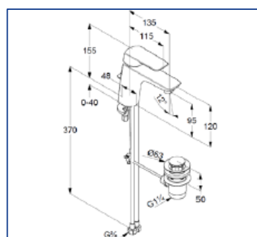
Schiță tehnică
