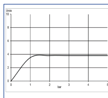
Diagramă debit
