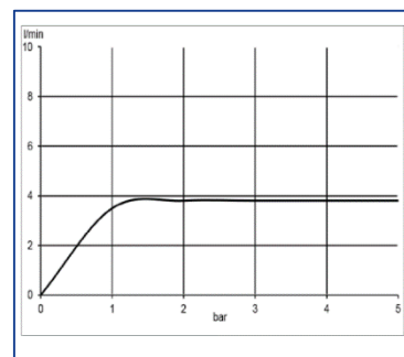
Diagramă debit
