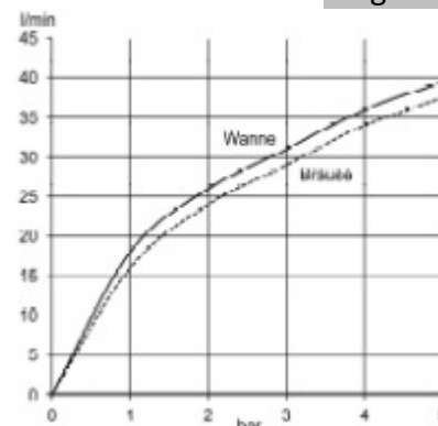
Diagramă debit
