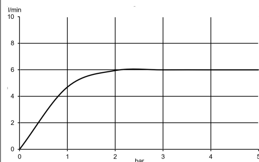
Diagramă debit
