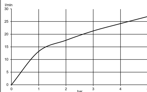
Diagramă debit
