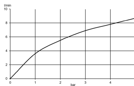
Diagramă debit
