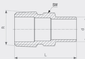
Übergangsstück - Rotguss Modell 94280G
