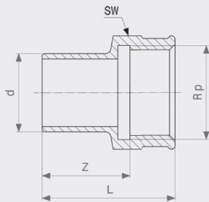
Einsteckstück - Rotguss Modell 94246G
