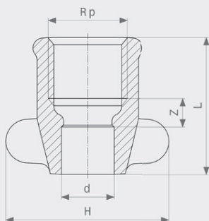
Übergangsstück - Rotguss Modell 94270GF
