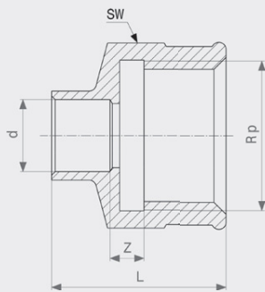
Übergangsstück - Rotguss Modell 94270G
