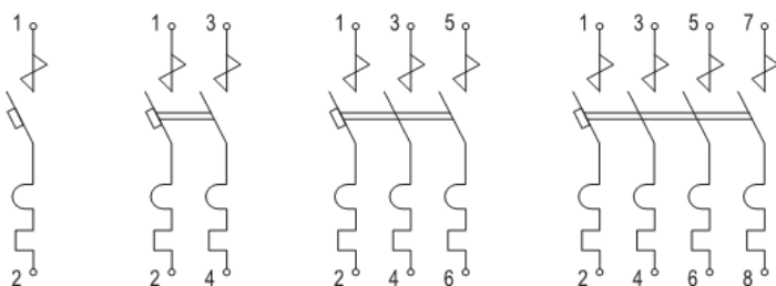
Fig.2 Schemele electrice
