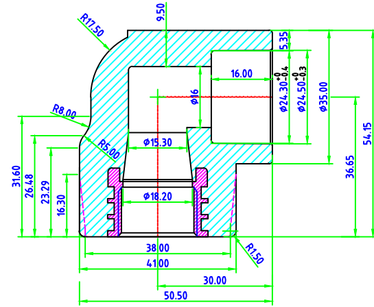
A-A KESİTİ
