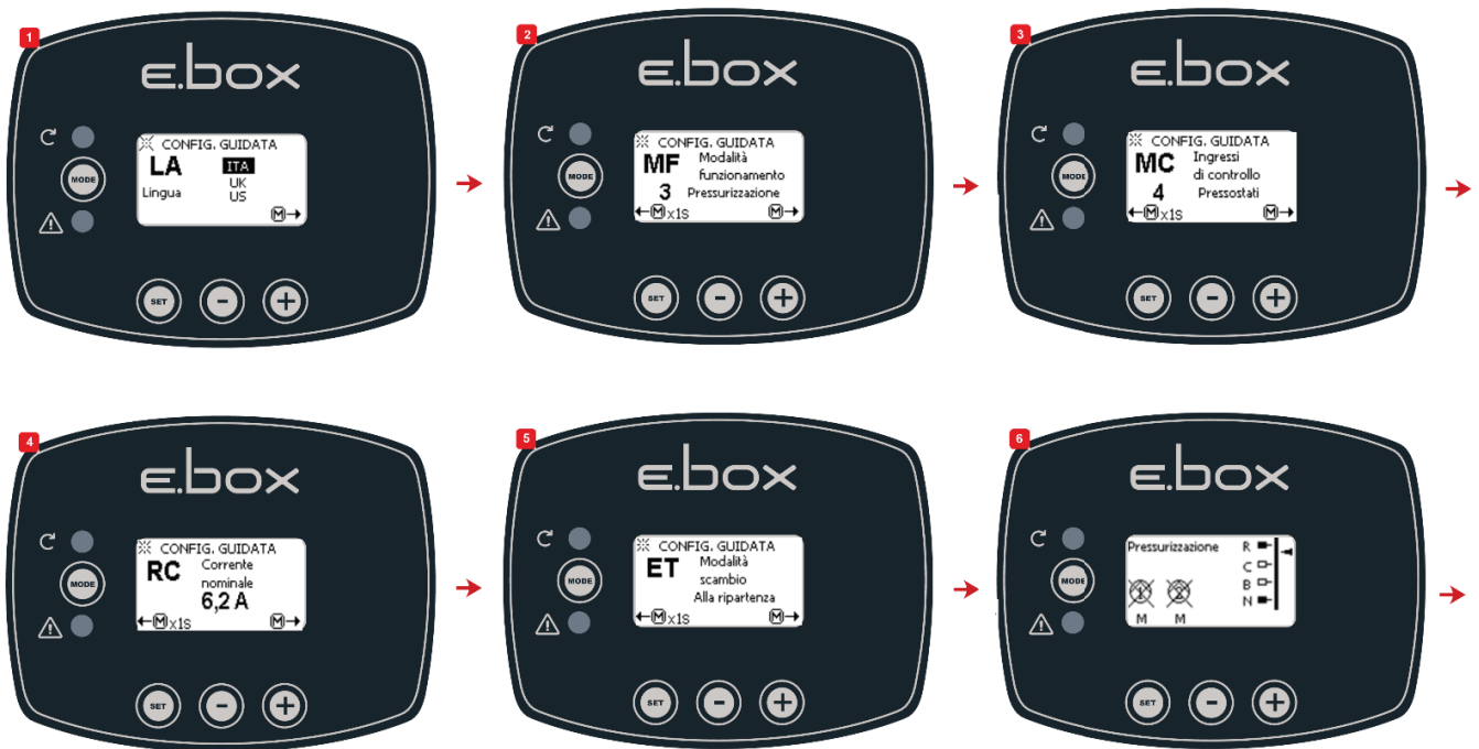
Figura 13: Configurare cu Presostați
