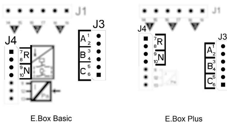
Figura 20: Intrări și protecții
