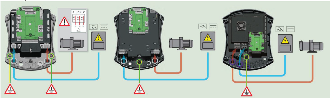
Figura 5: Conectări electrice
