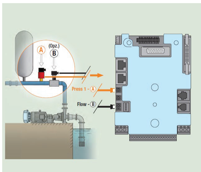
Figura 8: Conexiuni senzori
