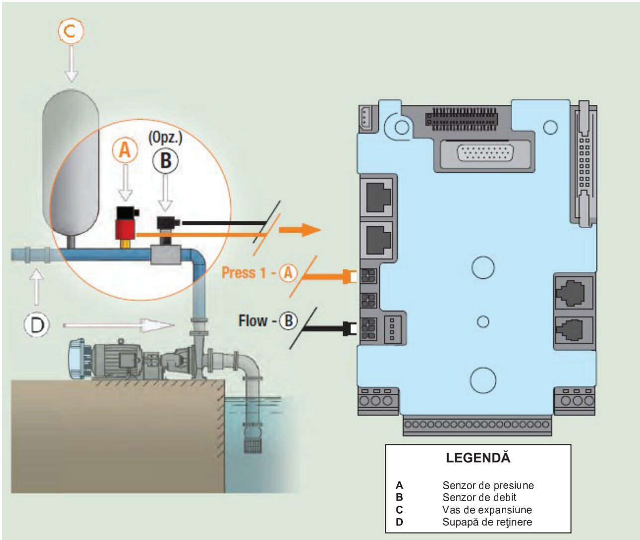
Figura 7: Instalația hidraulică
