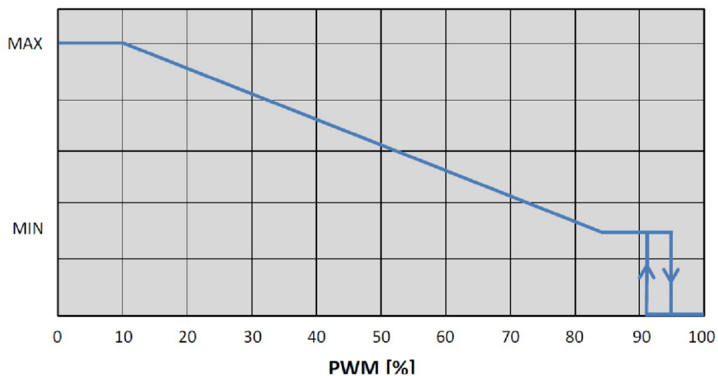
Profil PWM HEIZUNG
