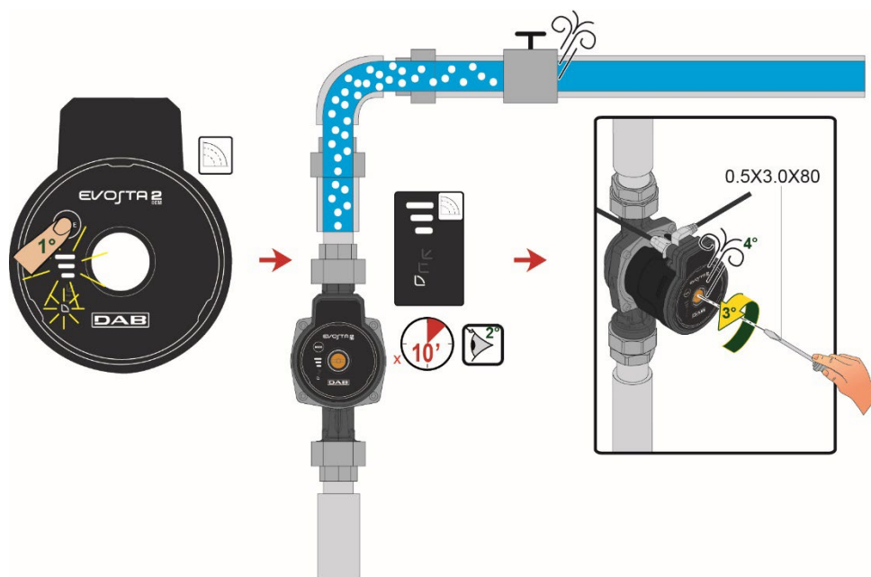
Obrázok 7: Odvzdušnenie čerpadla
