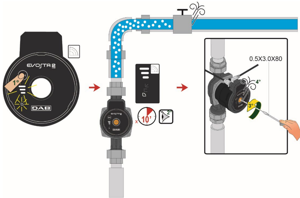
Kuva 7: Pumpun ilmaus
