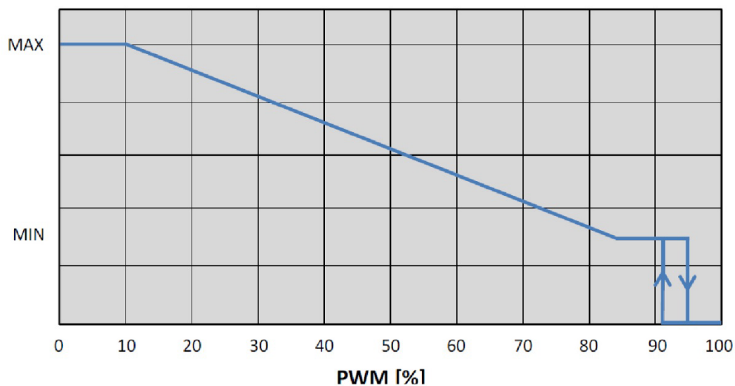
FŰTÉSI PWM profil
