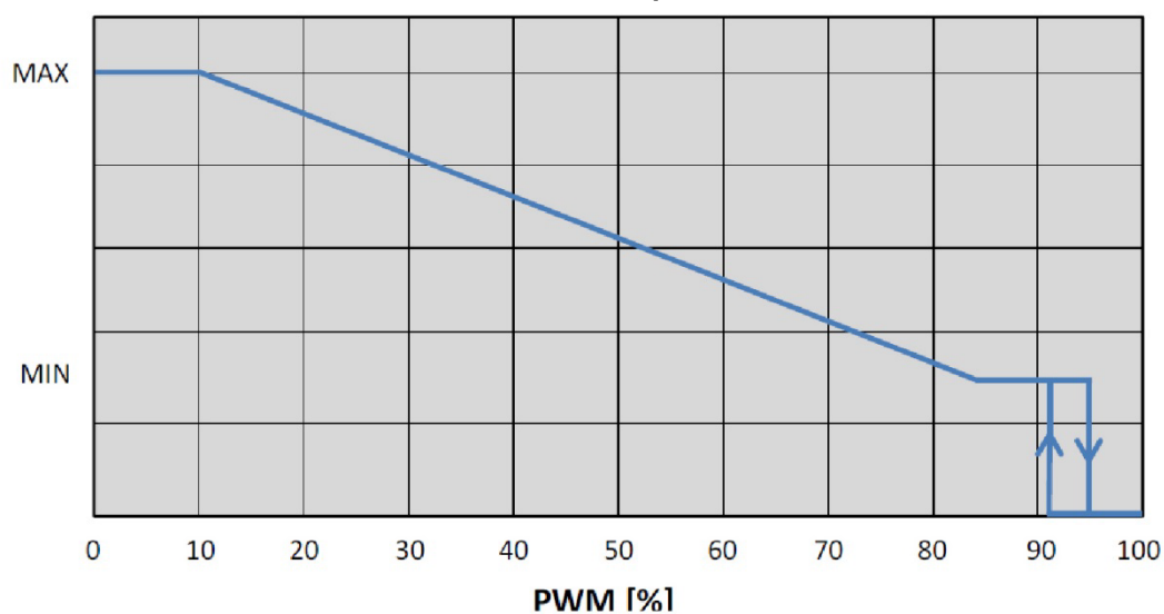
PWM ŠILDYMO profilis
