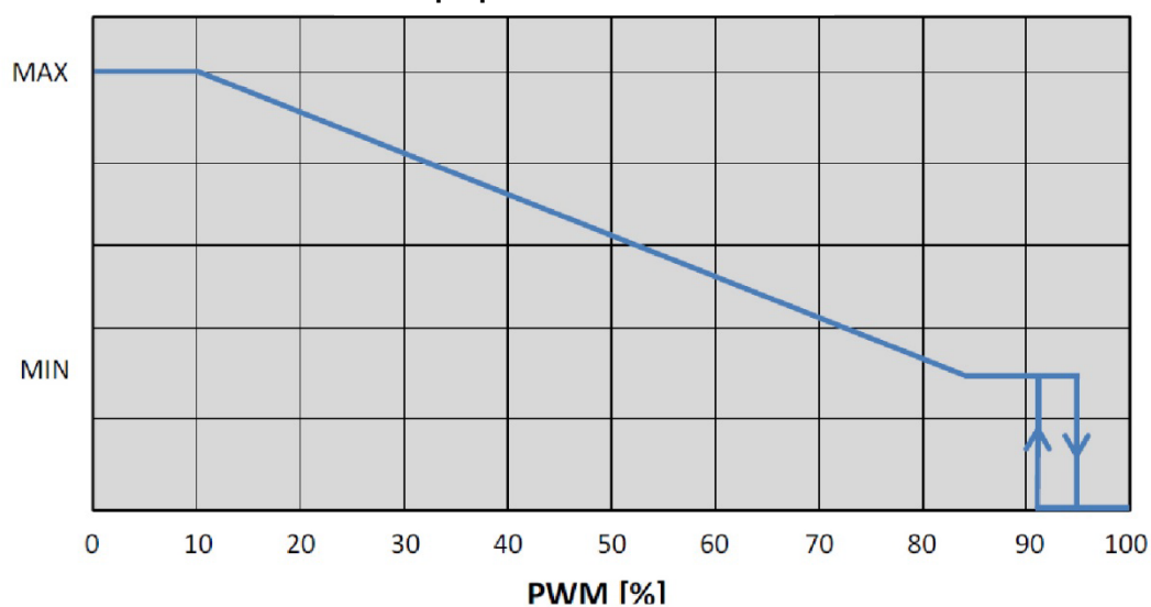
Профиль PWM НАГРЕВ
