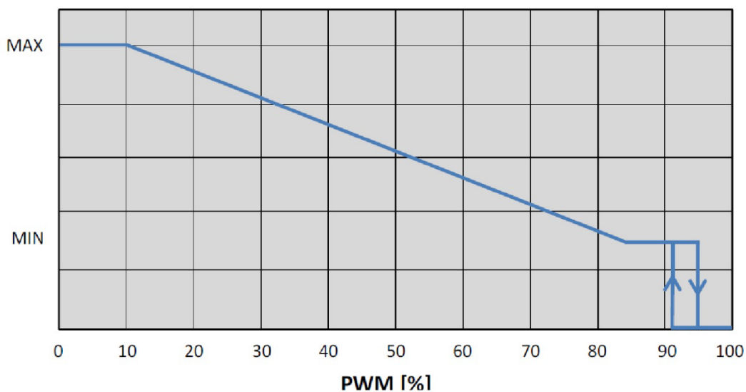
Προφίλ PWM ΘΕΡΜΑΝΣΗ
