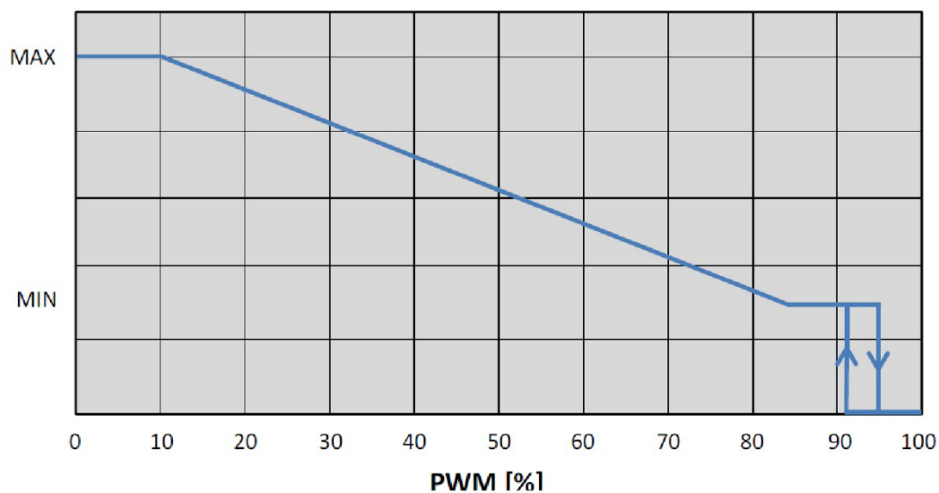
Profil PWM VYKUROVANIA
