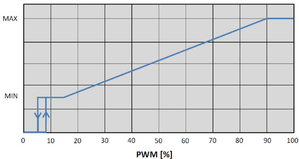
Profil PWM OGREVANJE
