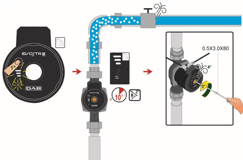
Figura 7: Aerisirea pompei
