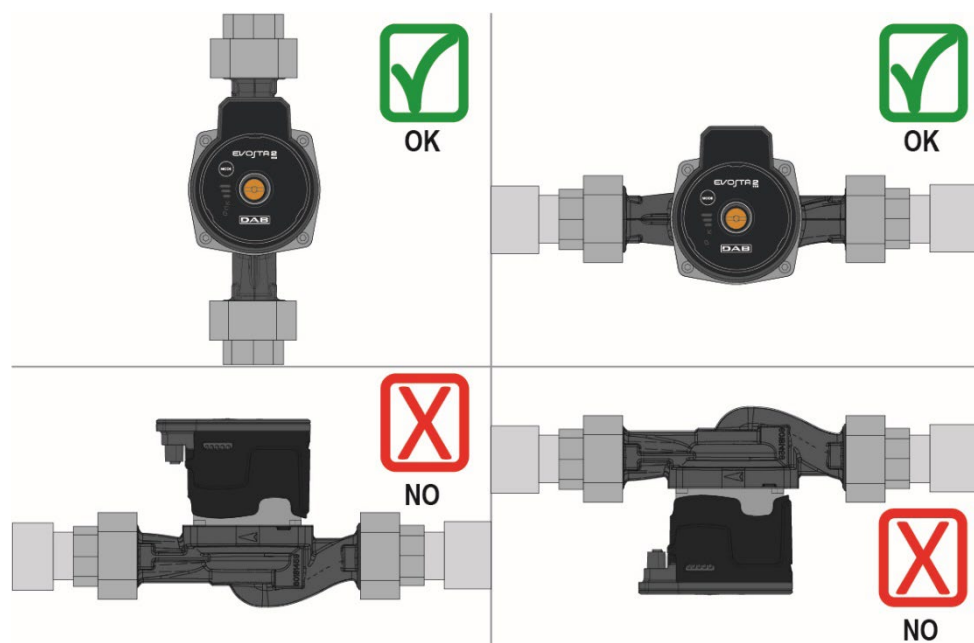
Obrázok 3: Montážna poloha
