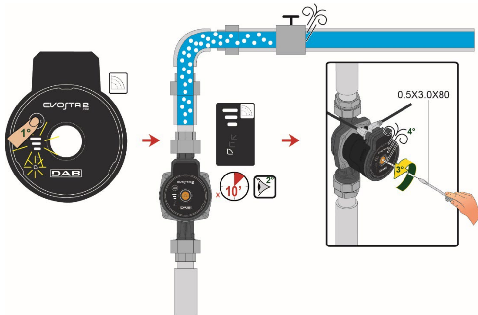
7. ábra: Pumpa légekiesztés
