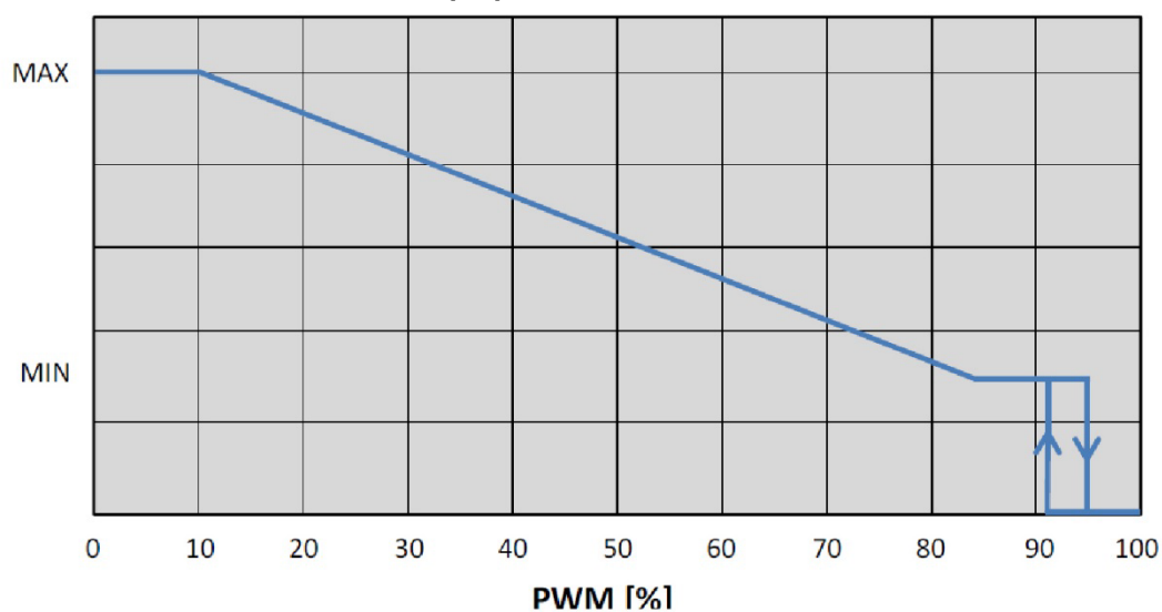
Профіль PWM НАГРІВ
