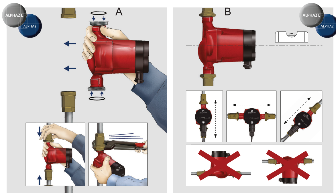
Fig. 3 Montajul GRUNDFOS ALPHA2 L
