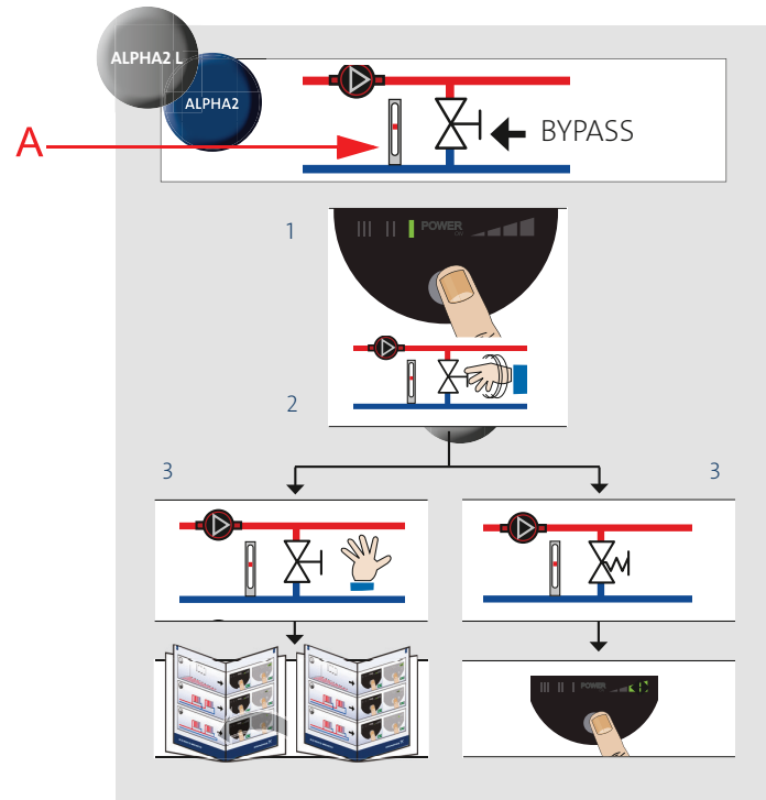
Fig. 10 Sisteme cu vană de ocolire
