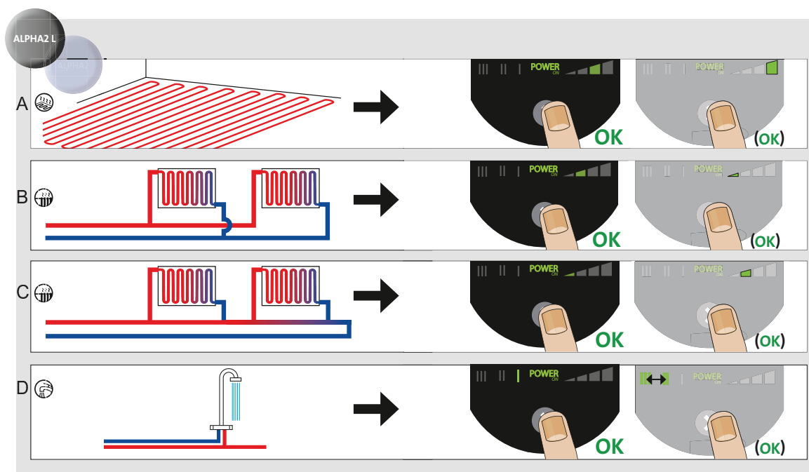
Fig. 9 Selectarea setării pompei pentru tipuri de sisteme
