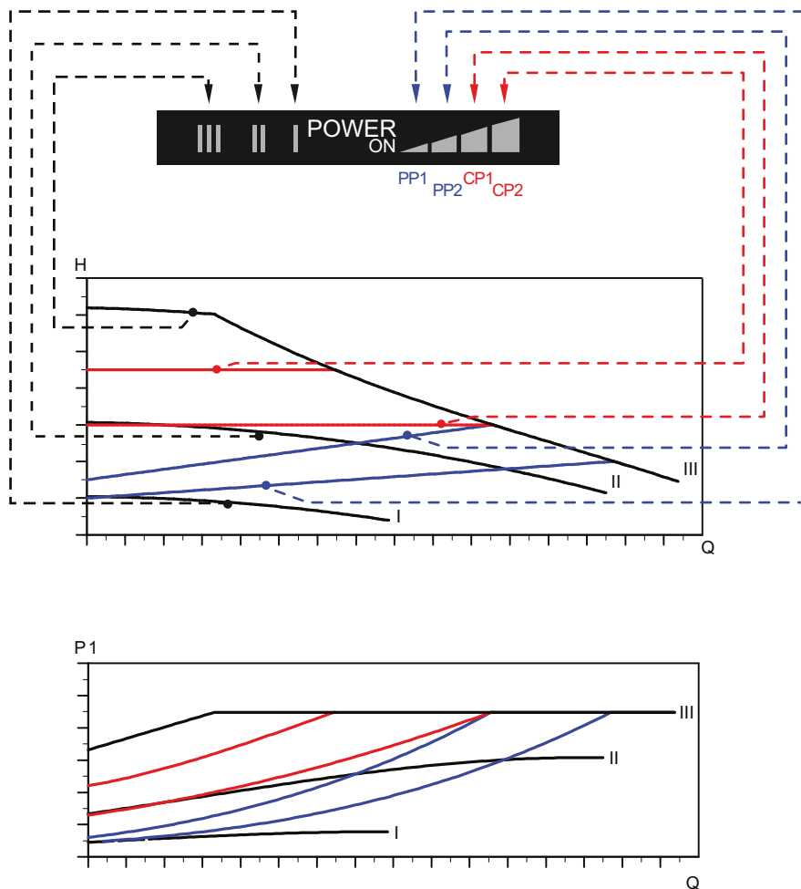
Fig. 17 Curbele caracteristice în funcție de setarea pompei
