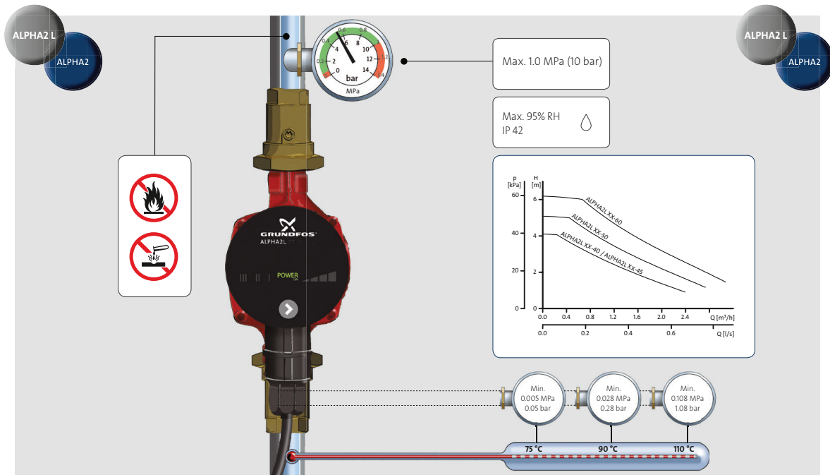
Fig. 2 Lichide pompate și condiții de exploatare
