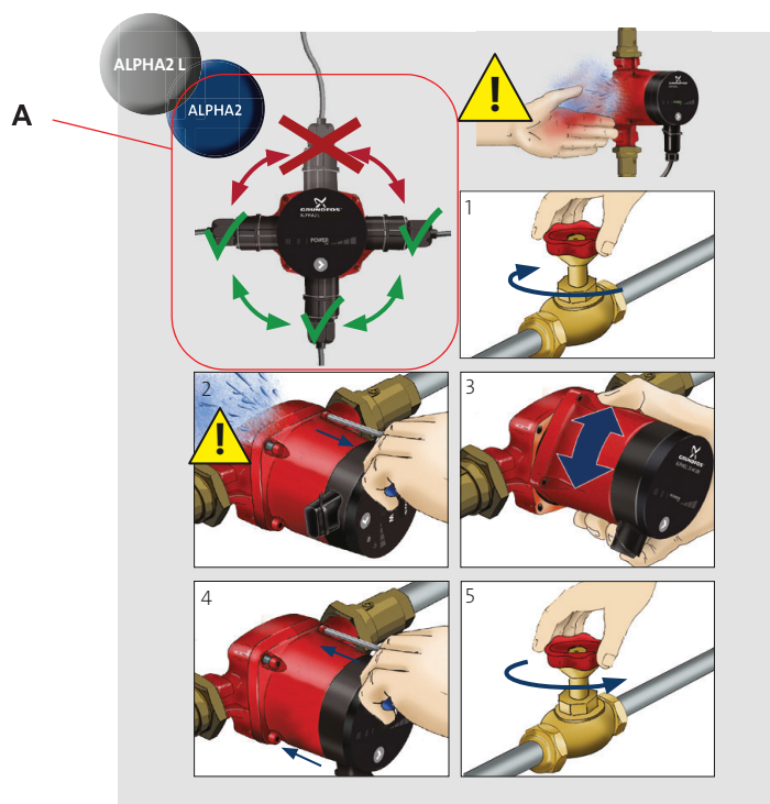
Fig. 4 Pozițiile cutiei de control
