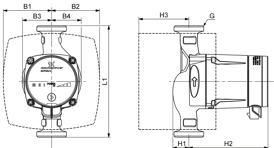
Fig. 14 Desene dimensionale, ALPHA2 L XX-40, XX-45, XX-50, XX-60
