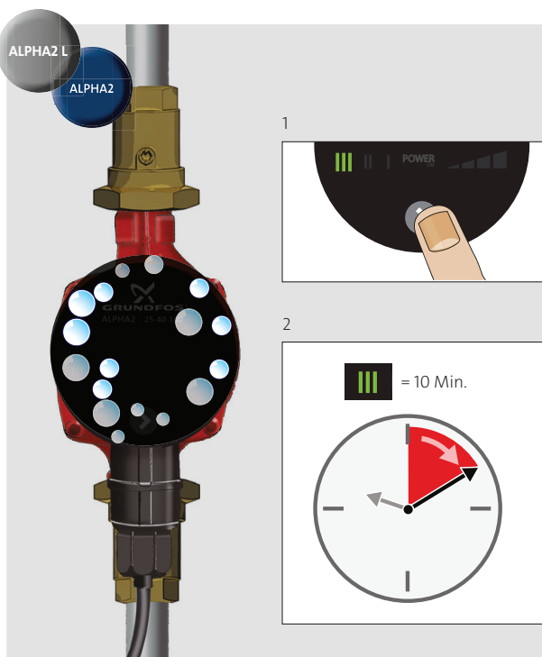
Fig. 11 Aerisirea pompei
