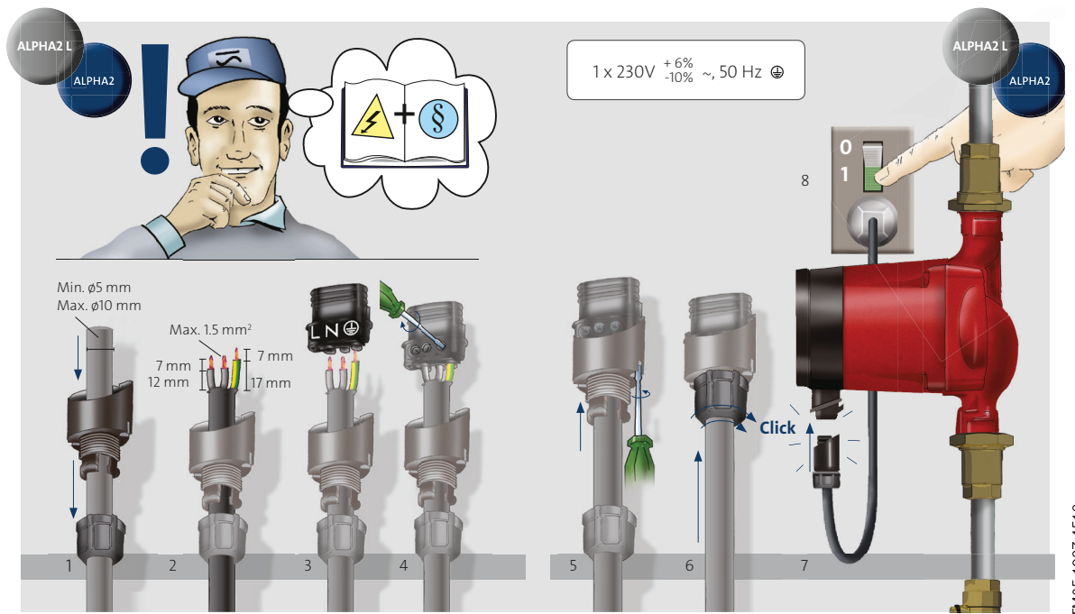
Fig. 6 Conexiunea electrică
