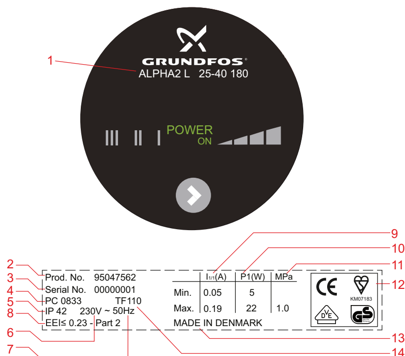
Fig. 22 Exemplu de plăcuță de identificare
