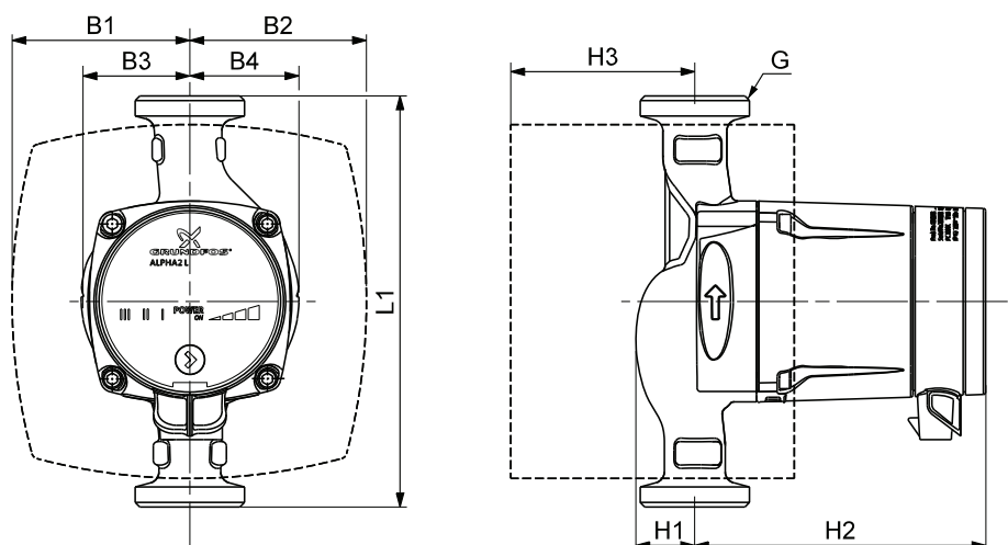
Fig. 15 Desene dimensionale, ALPHA2 L XX-40, XX-45, XX-60
