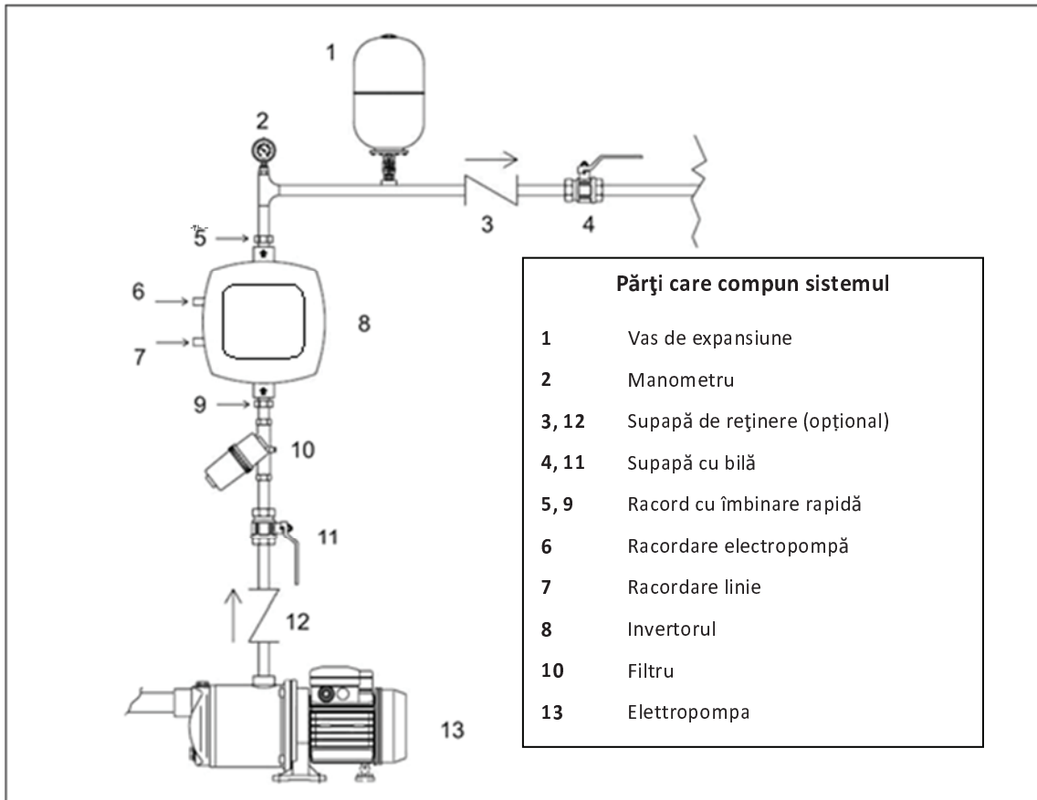
Figura 1: Instalație hidraulică
