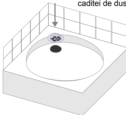
Fig.4 Pozitionarea si montarea scurgerii caditei de dus.
