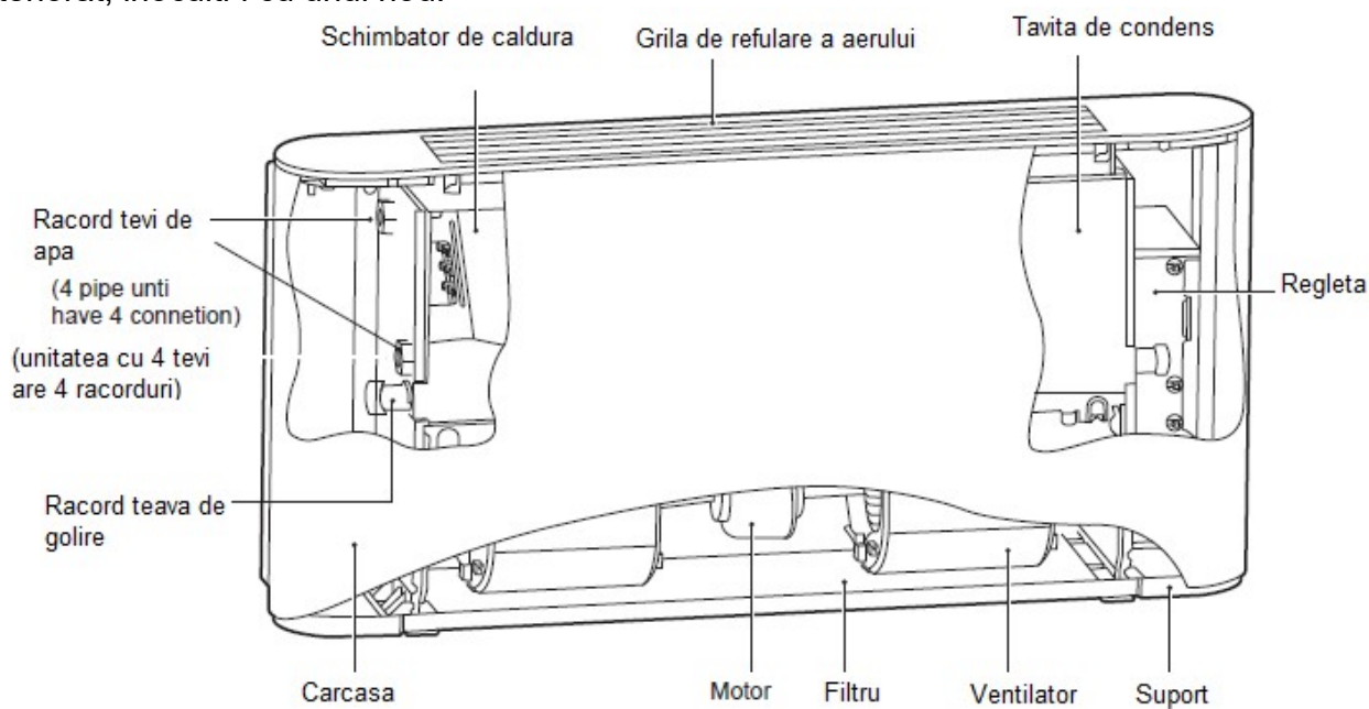
Figura 4-2 Schema unitatii cu montaj aparent
