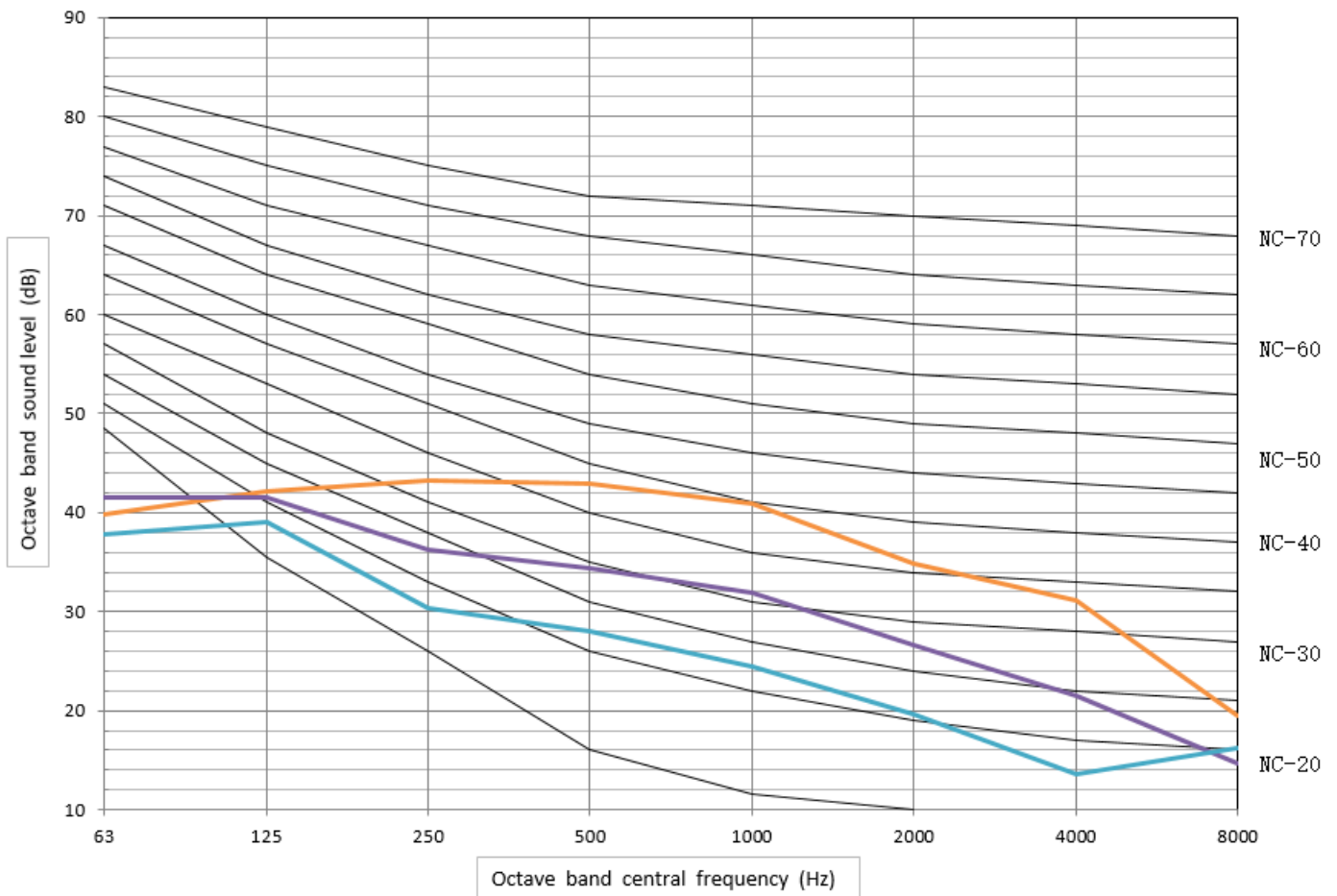
MKT4-800FG30-CL
