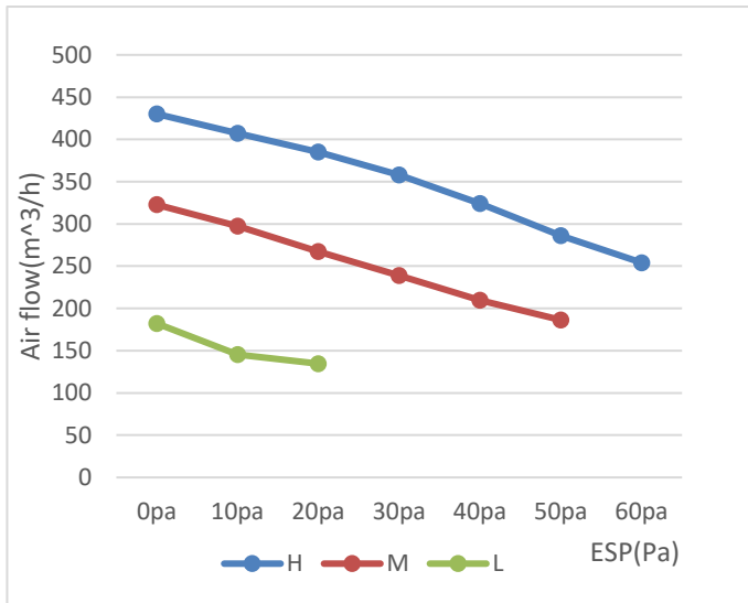
MKT4-200FG30-CL
