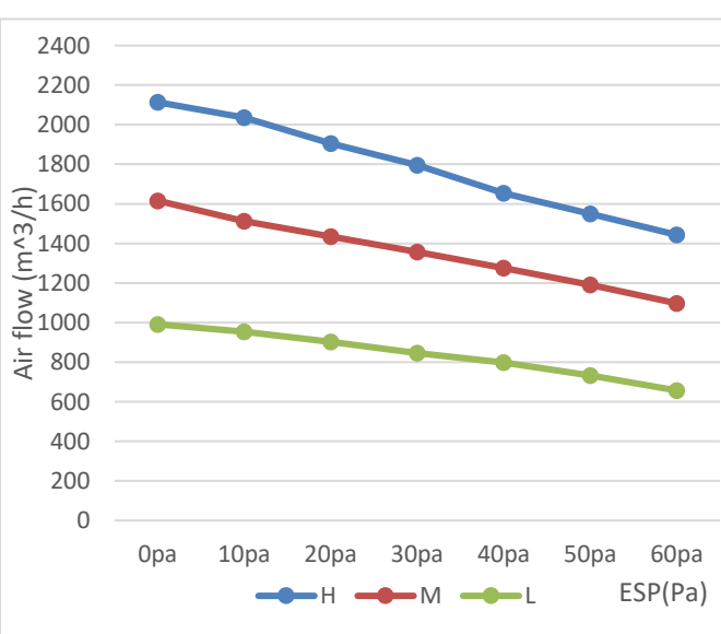
MKT4-1200FG30-CL
