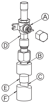
Ⓐ Kapama vanası Ⓑ Conta bölümü Ⓒ İç boru Ⓓ Çift gergi kısmı Ⓔ Bağlantı borusu Ⓕ Boru kapağı
