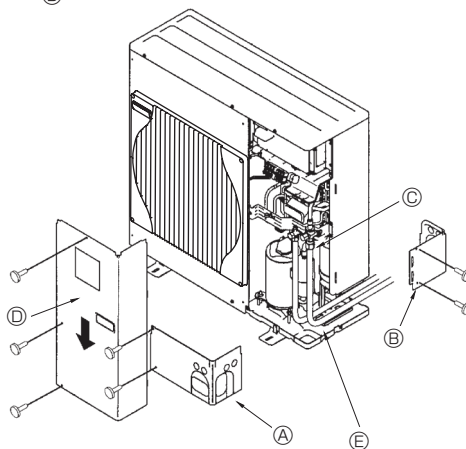
Ⓐ Deksel voorzijde Ⓑ Deksel achterzijde Ⓒ Afsluitkraan Ⓓ Onderhoudspaneel Ⓔ Buigstraal: 100 mm - 150 mm
