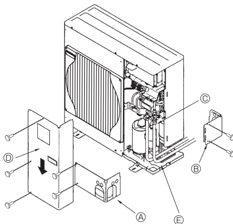
Ⓐ Vordere Leitungsabdeckung Ⓑ Leitungsabdeckung Ⓒ Absperrventil Ⓓ Wartungspult Ⓔ Radius der Biegung : 100 mm - 150 mm
