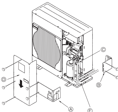
Ⓐ Panneau de protection avant Ⓑ Panneau de protection arrière Ⓒ Vanne d'arrêt Ⓓ Panneau de service Ⓔ Rayon de cintrage : 100 mm-150 mm
