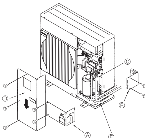
Ⓐ Cubierta de la tubería frontal Ⓑ Cubierta de la tubería posterior Ⓒ Válvula de parada Ⓓ Panel de servicio Ⓔ Radio del codo: 100 mm-150 mm
