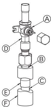
Ⓐ Vanne d'arrêt Ⓑ Côté joint d'étanchéité Ⓒ Tuyauterie locale Ⓓ Côté clé double Ⓔ Tuyau de jointure Ⓕ Gaine du tuyau
