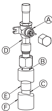
Ⓐ Válvula de retenção Ⓑ Secção de vedação Ⓒ Tubagem local Ⓓ Secção de chave dupla Ⓔ Tubo de junção Ⓕ Tampa do tubo
