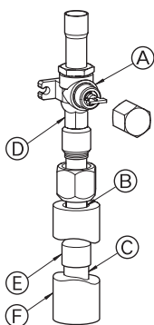
Ⓐ Afsluitkraan Ⓑ Afgedichte gedeelte Ⓒ Plaatselijke leiding Ⓓ Voor twee sleutels Ⓔ Verbindingspijp Ⓕ Pijpbedekking
