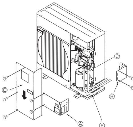
Ⓐ Lato anteriore pannello di copertura Ⓑ Lato posteriore pannello di copertura Ⓒ Valvola d'arresto Ⓓ Pannello di servizio Ⓔ Raggio della curva : 100 mm - 150 mm
