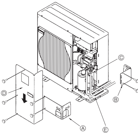
Ⓐ Ön kapak paneli Ⓑ Arka kapak paneli Ⓒ Kapama vanası Ⓓ Bakım paneli Ⓔ Şerit yarı çapı: 100 mm-150 mm
