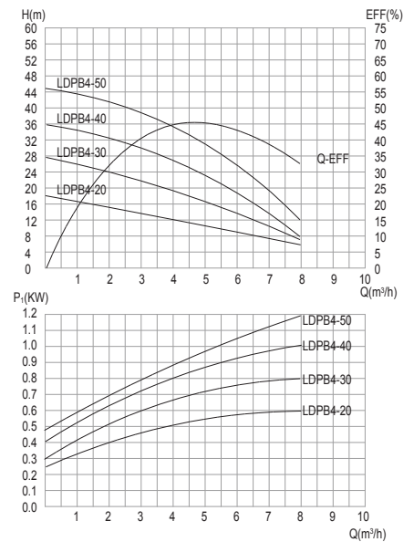
性能曲线图 (Performance Curves)
