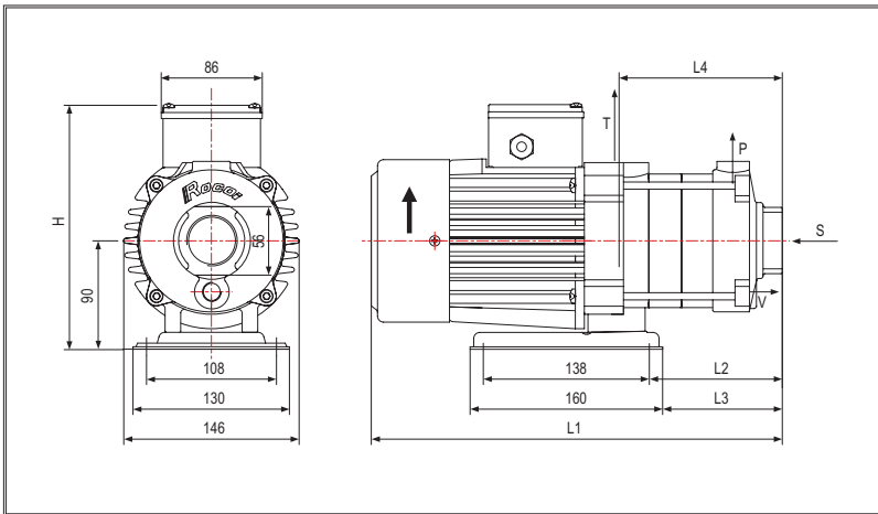
外形图 (Outline Drawing)
