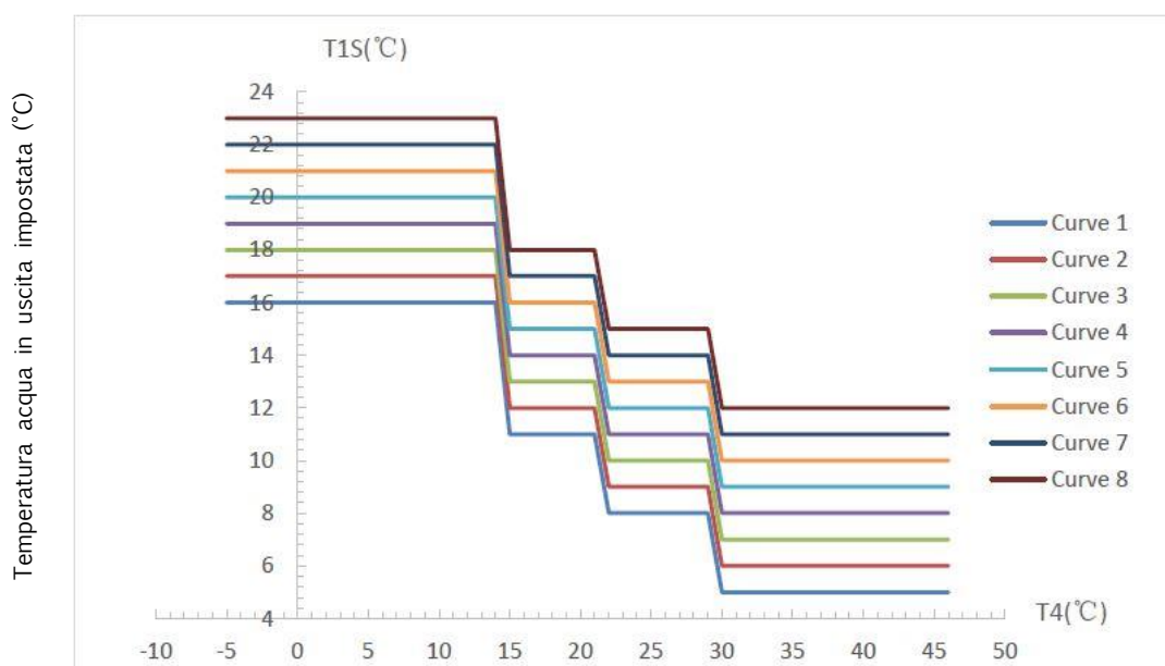
Curve di bassa temperatura per il modo Raffreddamento
